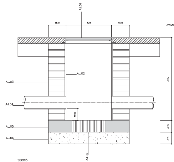
AJ. INSTAL·LACIONS COMPLEMENTÀRIES DE PREVISIÓ PERICÓ REGISTRE INSTAL·LACIONS
