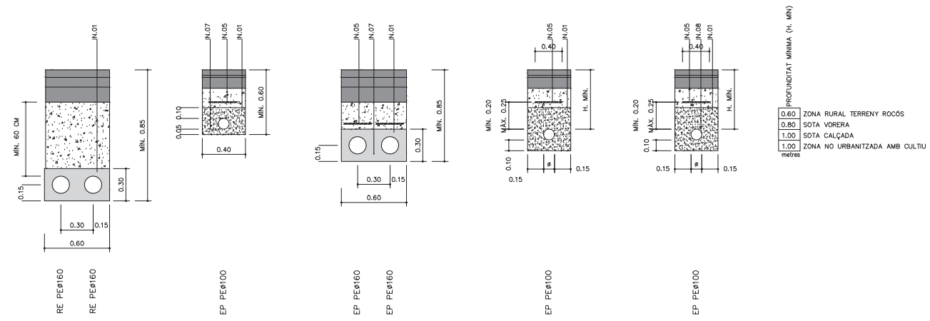
RE. TUBS DE RESERVA EP. ENLLUMENAT PÚBLIC G. XARXA DE GAS
