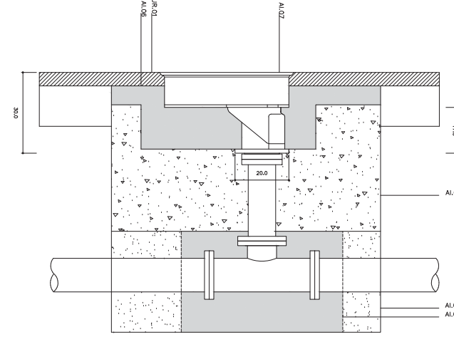
PERICÓ HIDRANT D'INCENDIS
