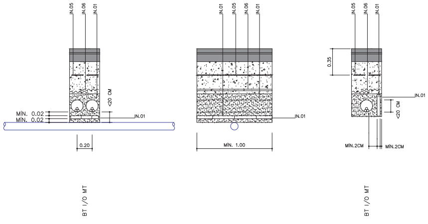
CREUAMENT AMB ALTRES SERVEIS PER SOTA DISTÀNCIA MÍNIMA
