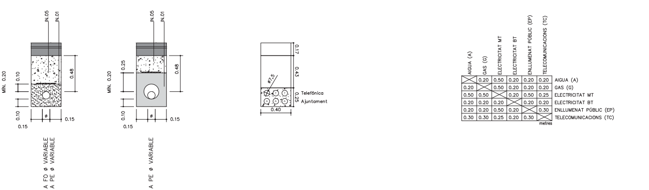
A. XARXA D'AIGUA POTABLE I D'HIDRANTS D'INCENDI TC. XARXA DE TELECOMUNICACIONS
