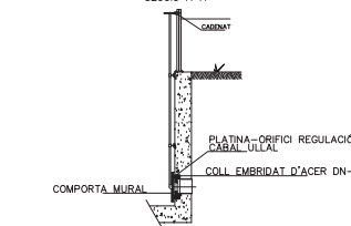
INSTAL·LACIÓ COMPORTA MURAL I ACCESSORIS REGULACIÓ CABAL UL·LAL SECCIÓ A-A'
