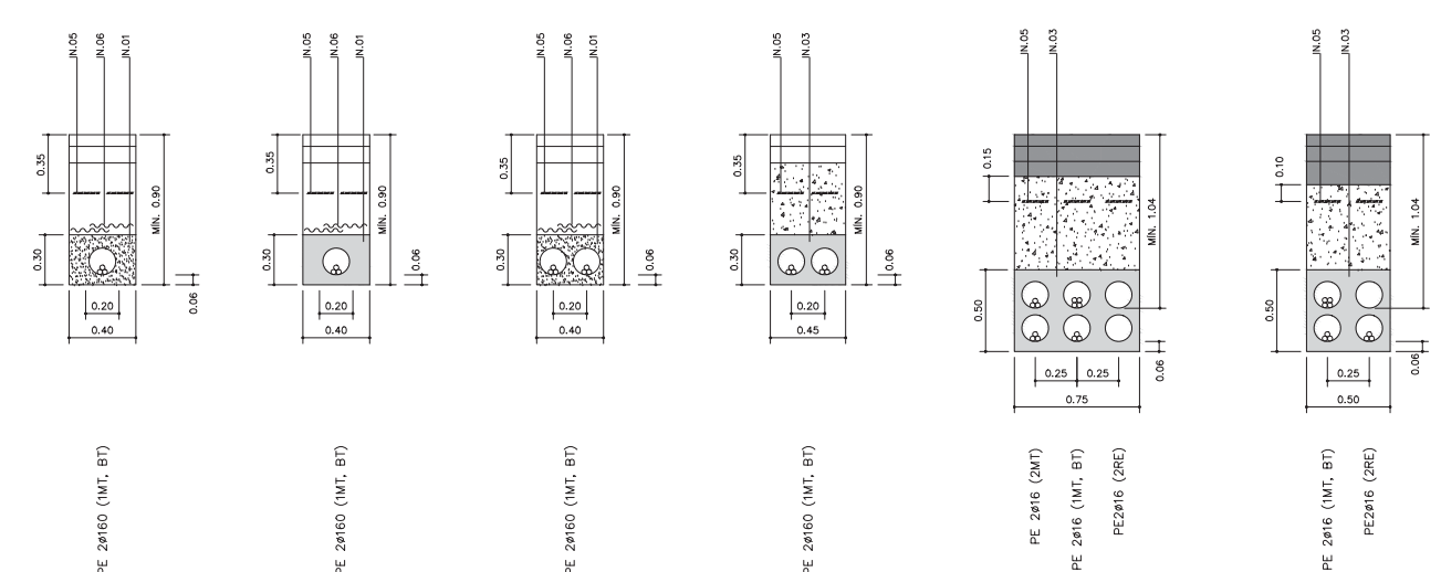
MT, BT, RE. XARXA ELÈCTRICA SOTERRADA DETALLS TIPUS DE LES XARXES DE SERVEIS INDIVIDUALITZADES
