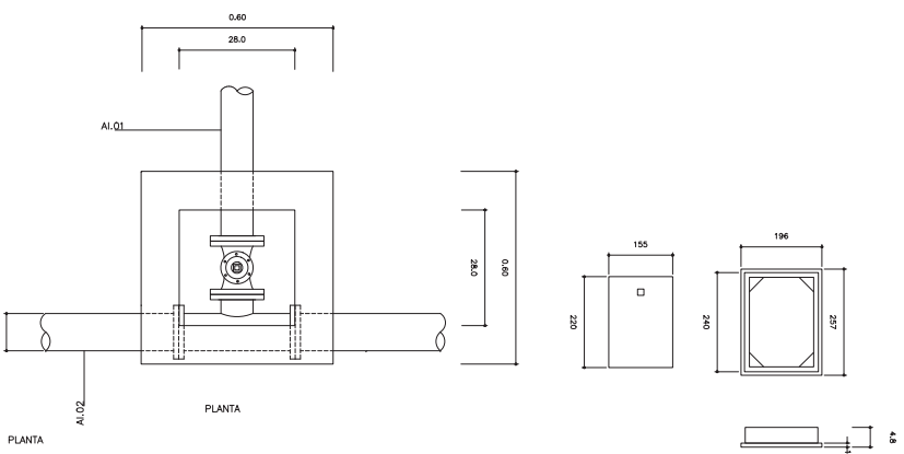
SE. SÈQUIA INSTAL·LACIÓ COMPORTA SÈQUIA
