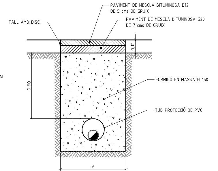
CREUAMENT VIAL EN ZONA JA PAVIMENTADA PER A CONDUCCIONS DE POLIETILE
