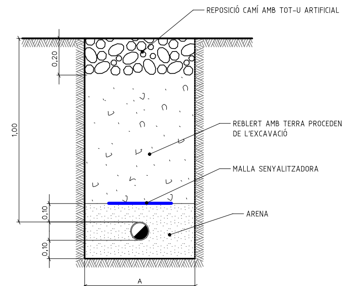
RASA TIPUS PER A CAMINS EN ZONA NO URBANITZADA I RUSTICA
