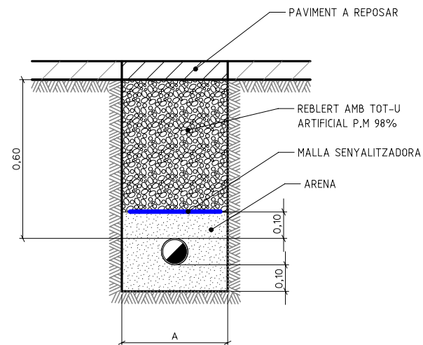
RASA TIPUS EN VORERA ZONA URBANA
