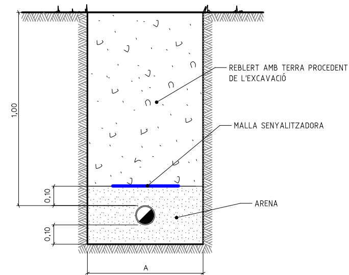
RASA TIPUS EN ZONA NO URBANITZADA I RUSTICA
