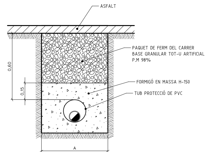
CREUAMENT VIAL EN OBRA D'URBANITZACIO PER A CONDUCCIONS DE POLIETILE
