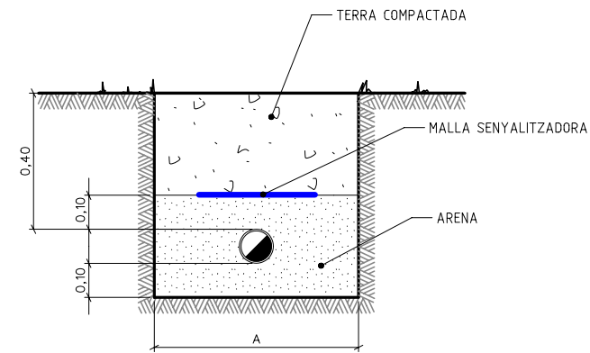
RASA TIPUS EN ROCA
