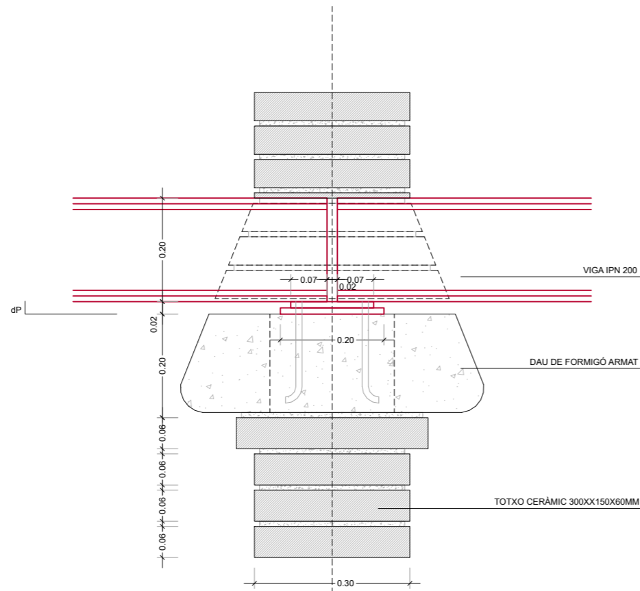
DETALL SECCIÓ 01 - ALÇAT CAPITELL PILAR e1/10
