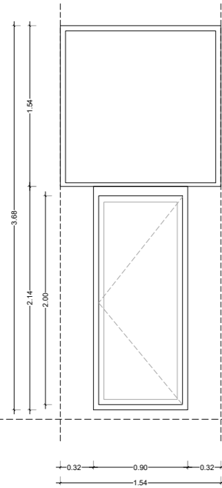
PROPOSTA FUSTERIA - F01
