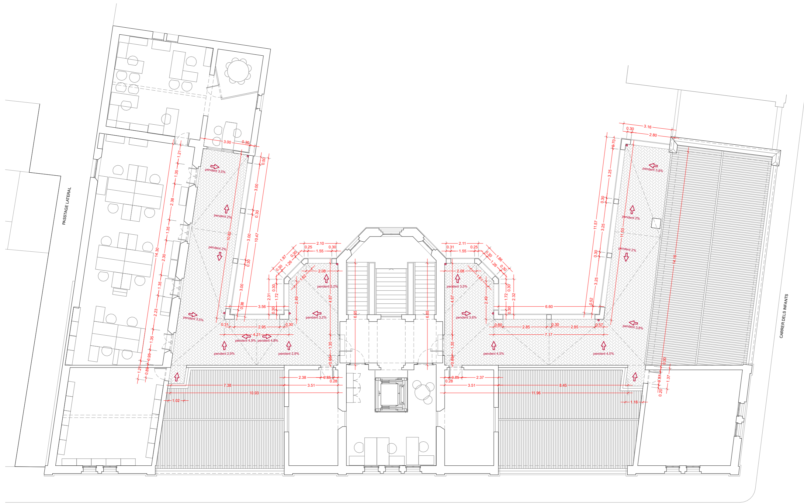
P2. PLANTA EDIFICI INFANTS - PLANTA SEGONA
