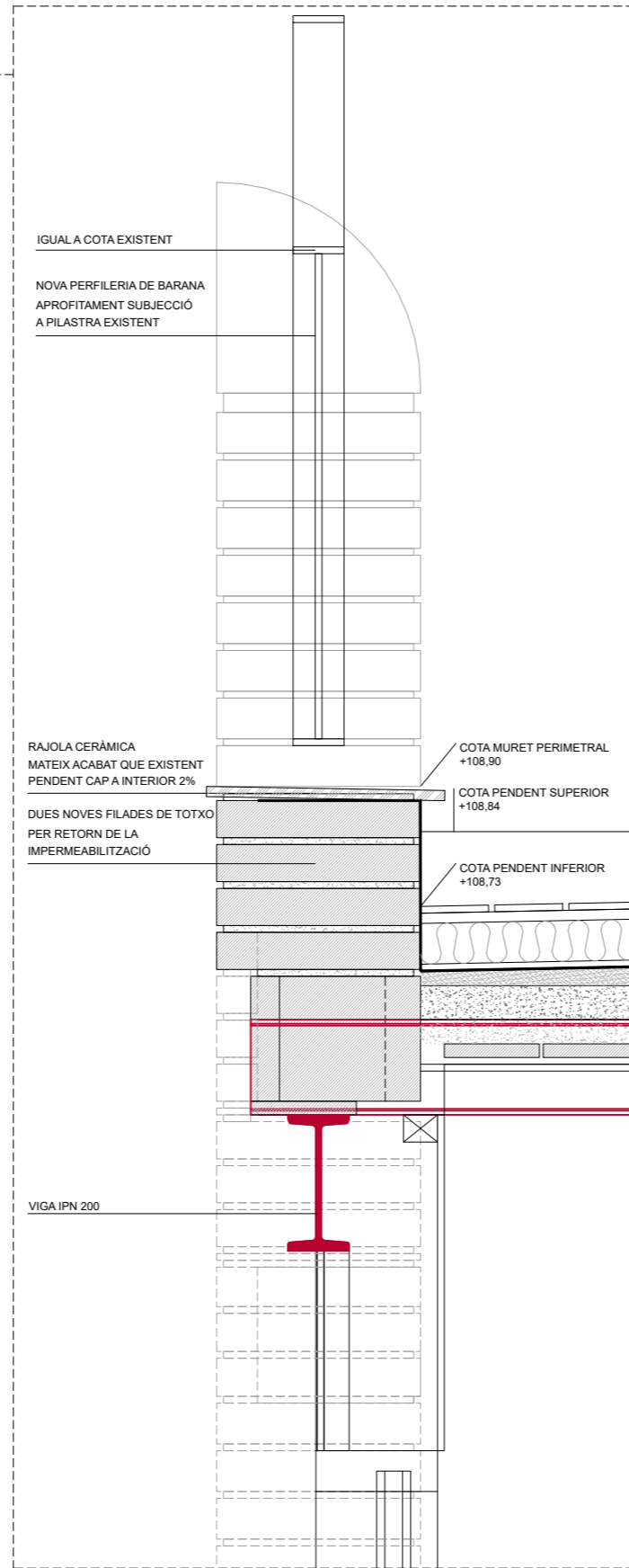
DETALL TROBADA FAÇANA-COBERTA e1/10
