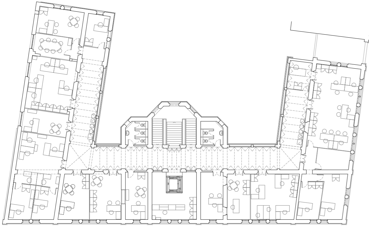
P1. PLANTA EDIFICI INFANTS - PLANTA PRIMERA
