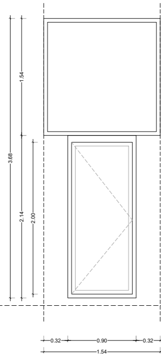
PROPOSTA FUSTERIA - F04
