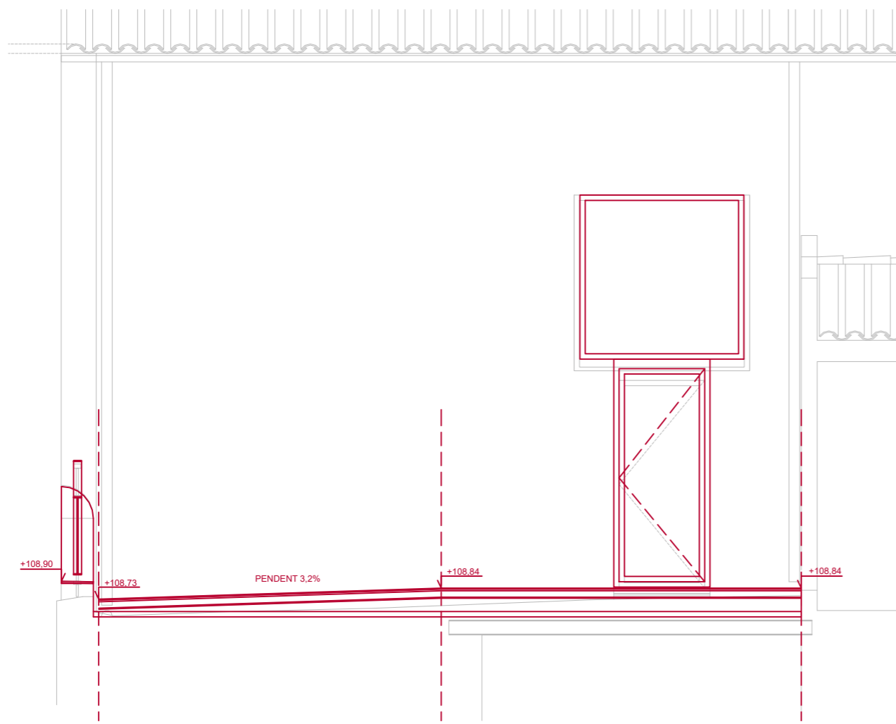
SD. SECCIÓ TERRAT
