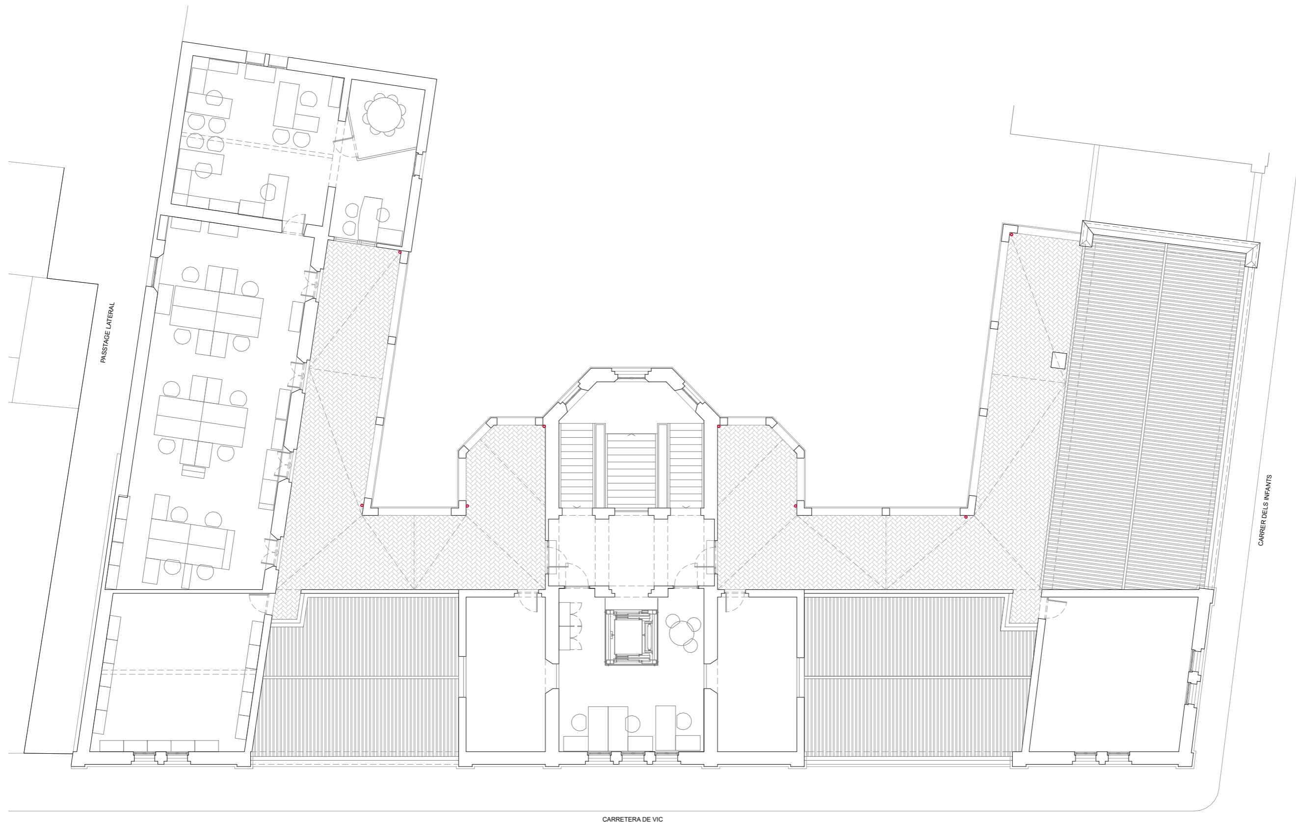
P2. PLANTA EDIFICI INFANTS - PLANTA SEGONA
