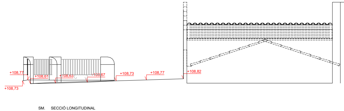
SM. SECCIÓ LONGITUDINAL
