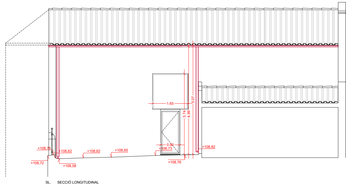
SL. SECCIÓ LONGITUDINAL
