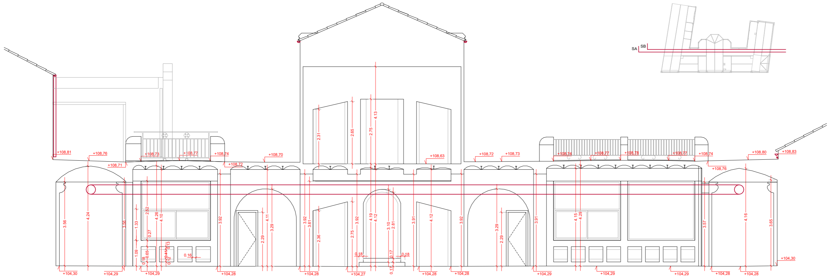
SB. SECCIÓ LONGITUDINAL
