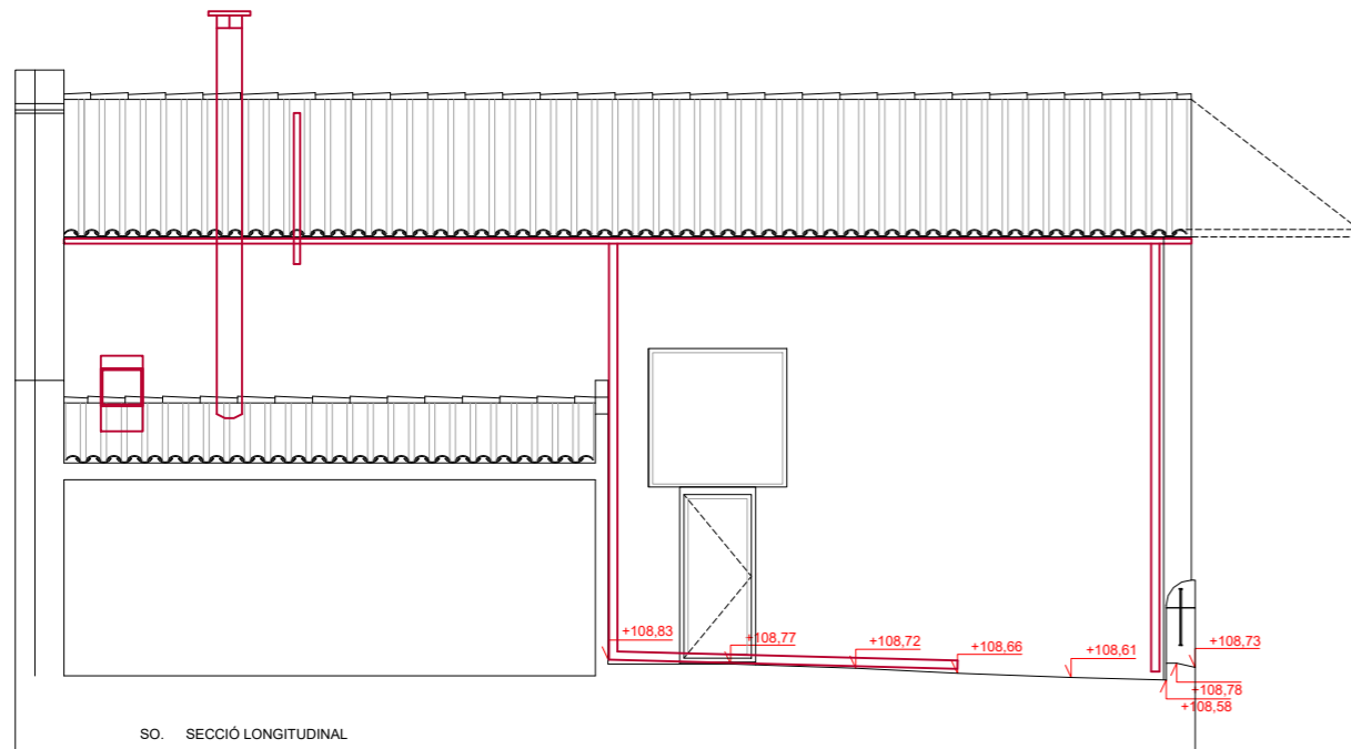
SO. SECCIÓ LONGITUDINAL
