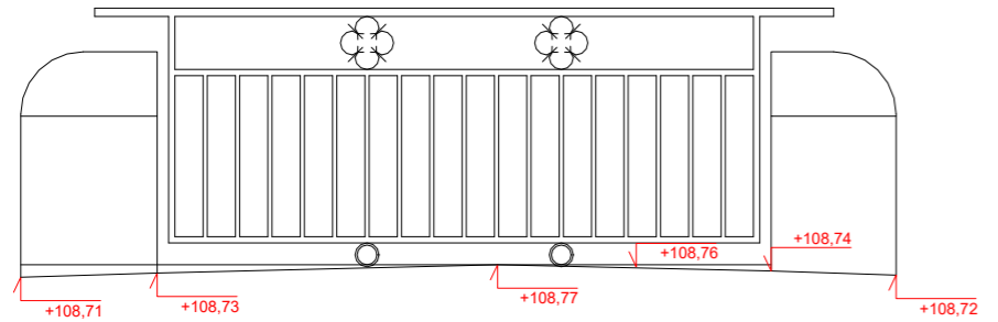
A04. ALÇAT TRAM 04
