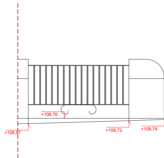
B03. ALÇAT TRAM 03
