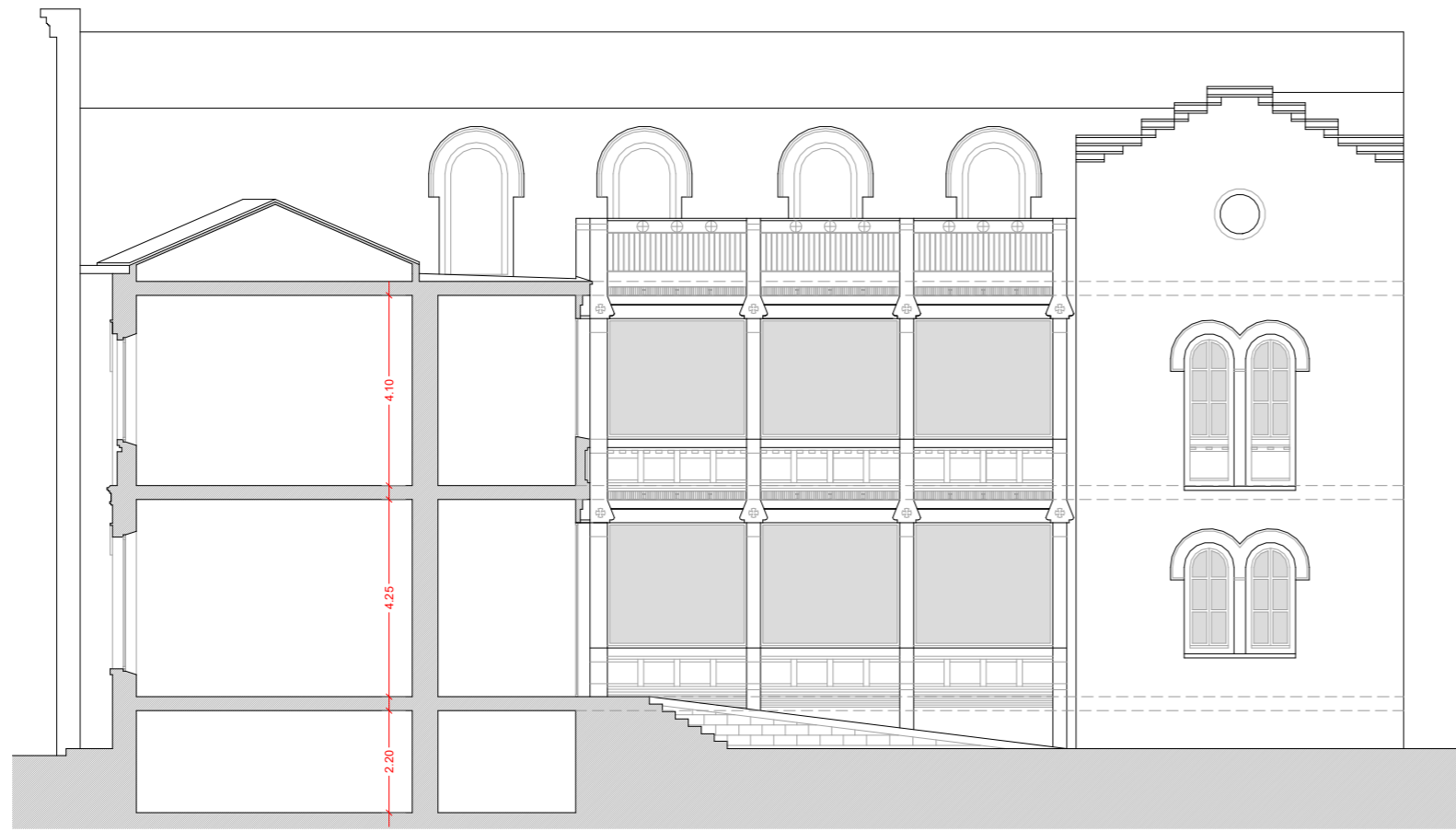
S1. SECCIÓ GENERAL PATI INTERIOR 1
