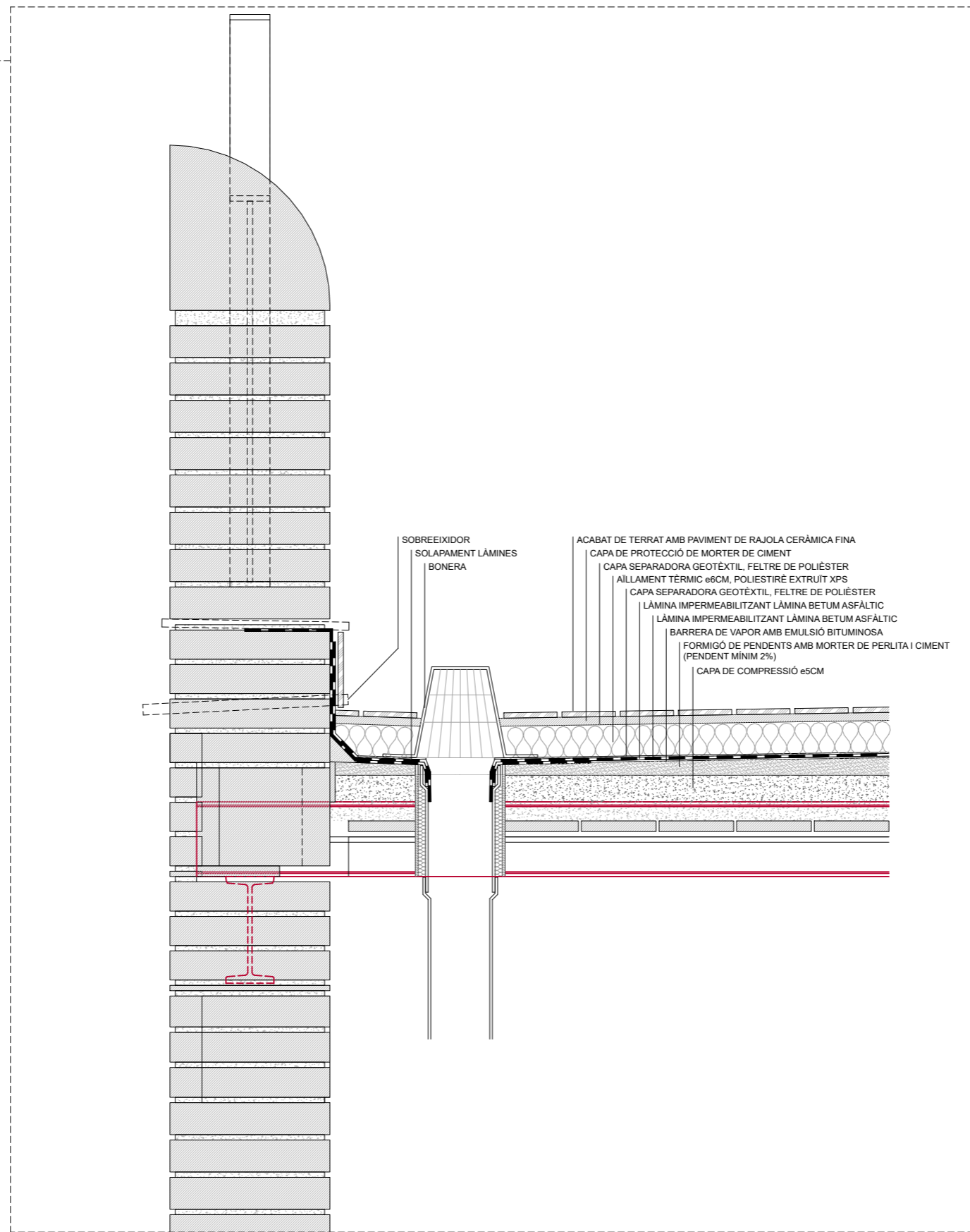
DETALL TROBADA BONERA e1/10
