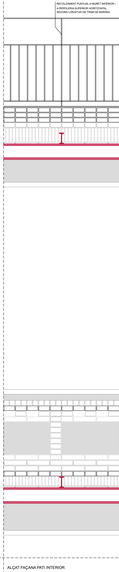
ALÇAT FAÇANA PATI INTERIOR e1/30
