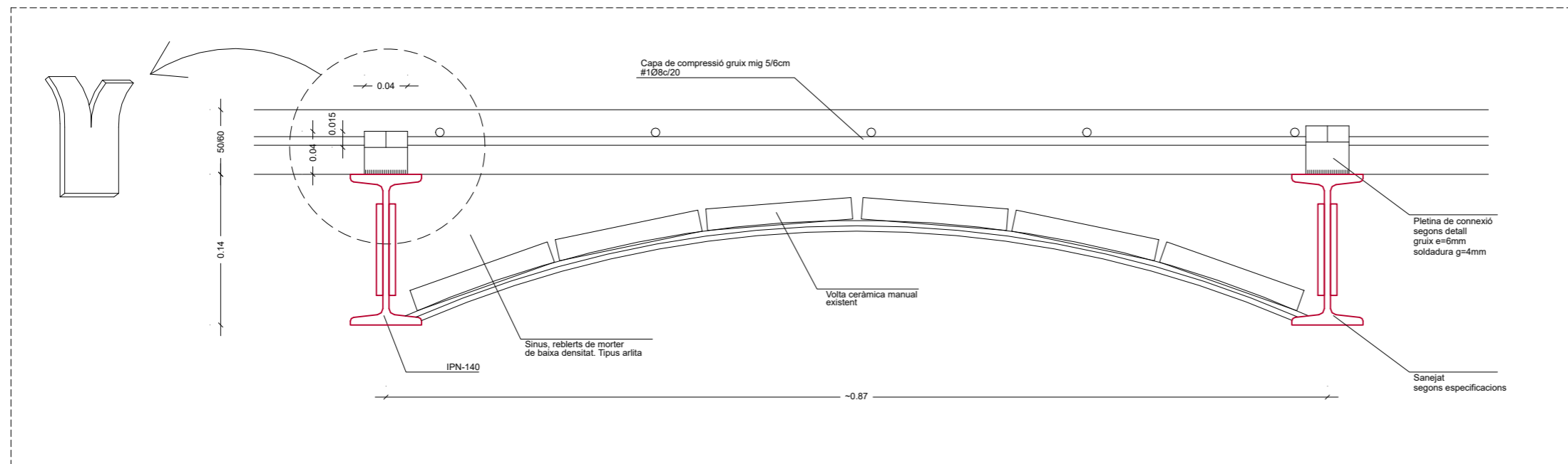
SECCIÓ REFORÇADA e1/5
