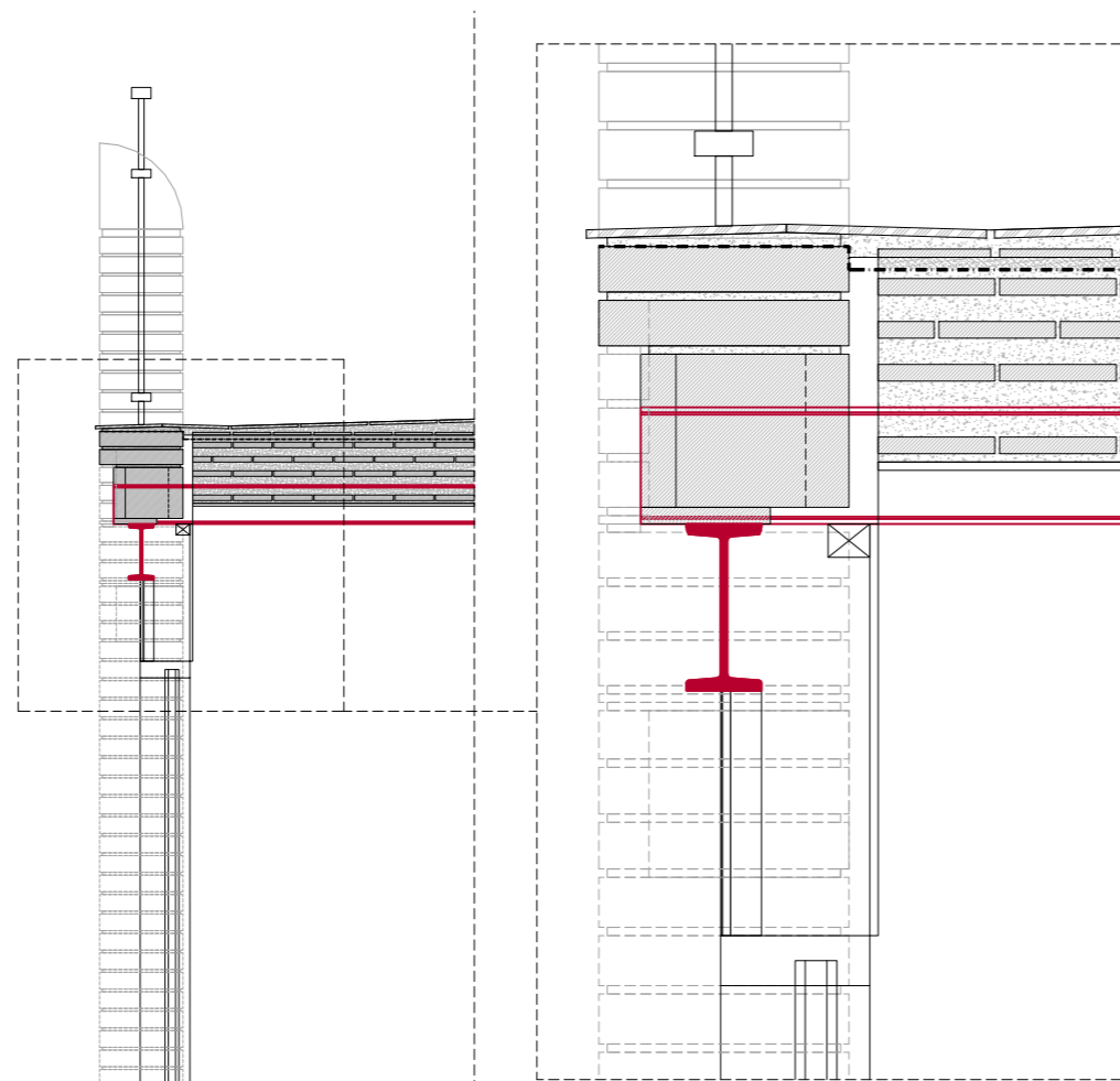
DETALL TROBADA FAÇANA-COBERTA e1/10
