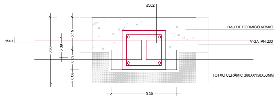
DETALL PLANTA CAPITELL PILAR e1/10
