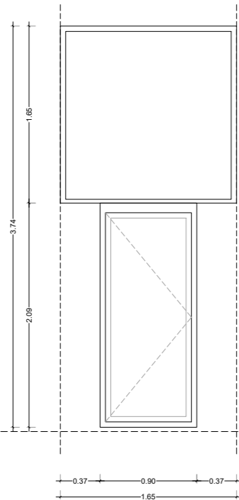
ESTAT ACTUAL FUSTERIA - F04
