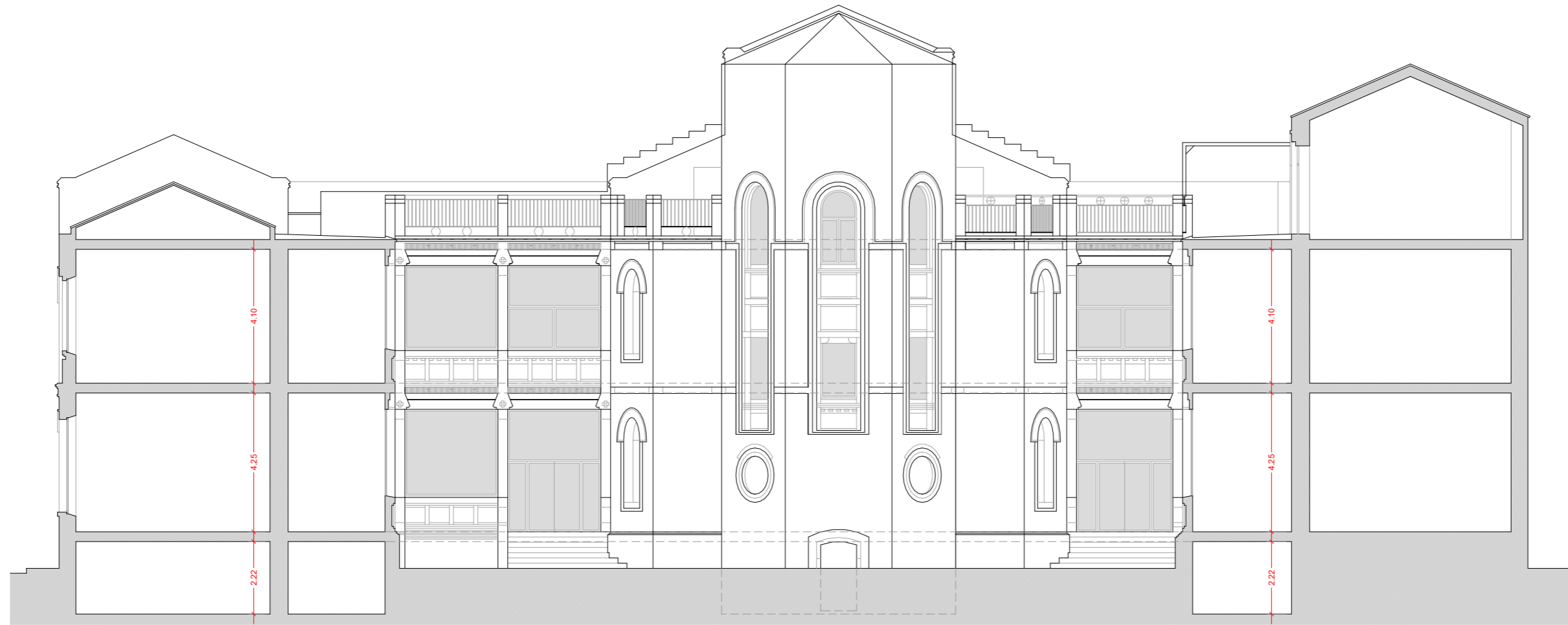
S2. SECCIÓ GENERAL PATI INTERIOR 2
