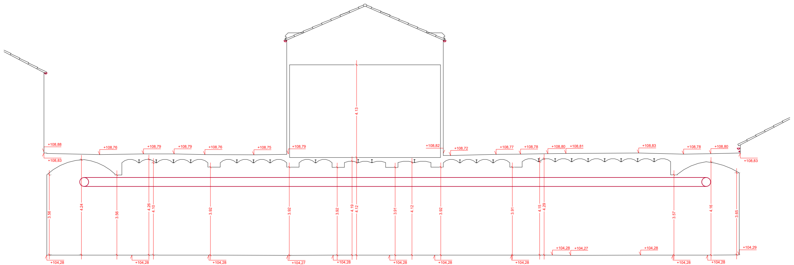
SA. SECCIÓ LONGITUDINAL
