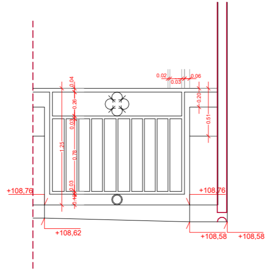
A01. ALÇAT TRAM 01
