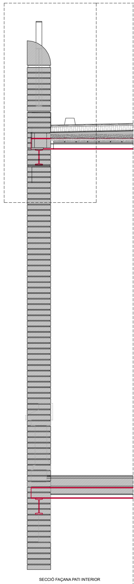
SECCIÓ FAÇANA PATI INTERIOR e1/30
