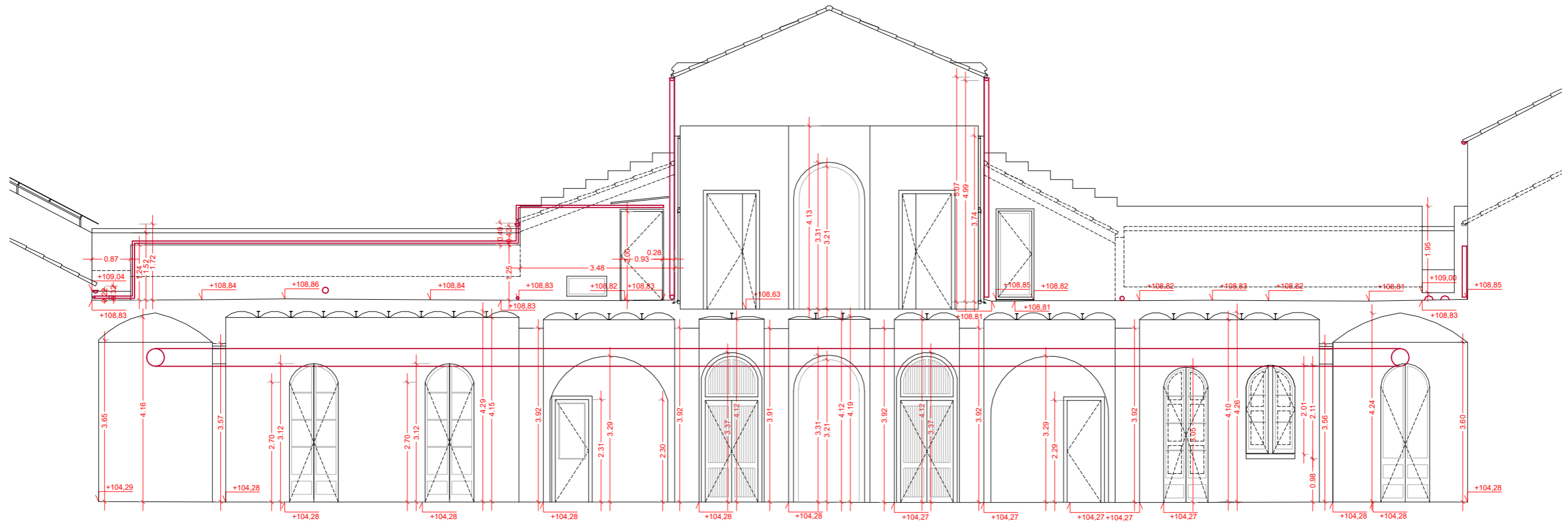
SC. SECCIÓ LONGITUDINAL
