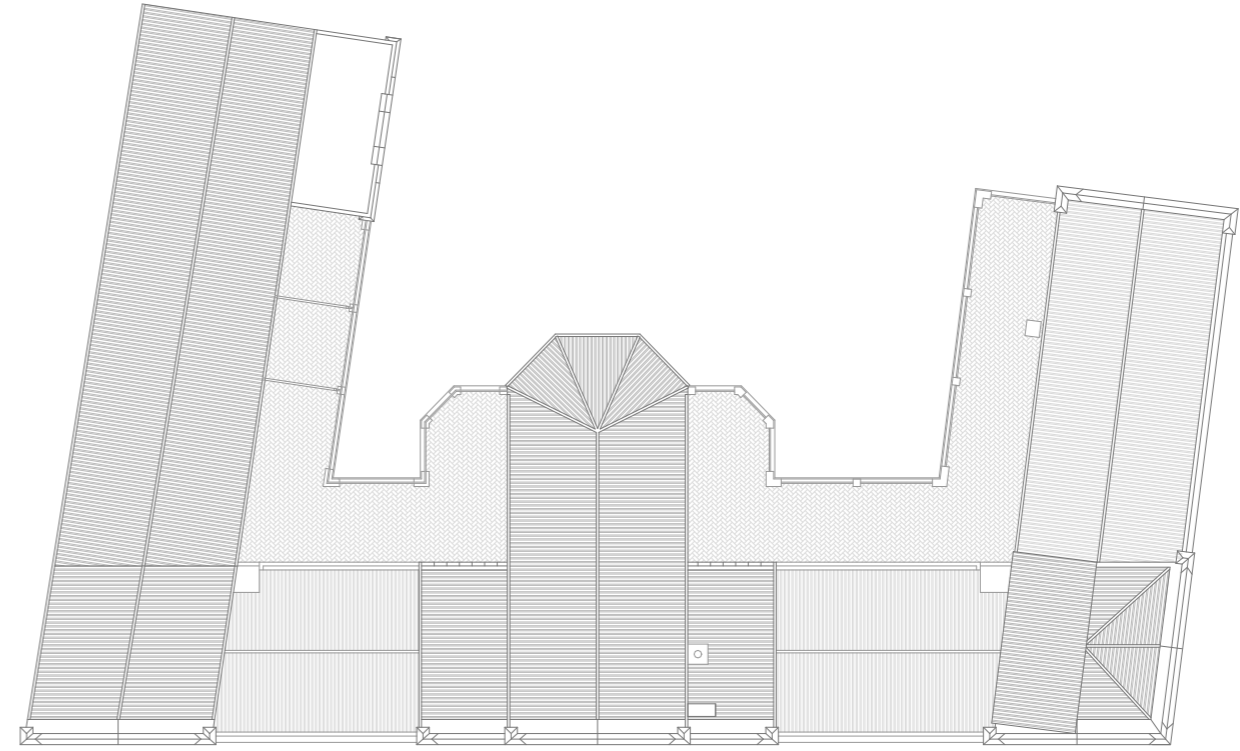
PC. PLANTA EDIFICI INFANTS - PLANTA COBERTA
