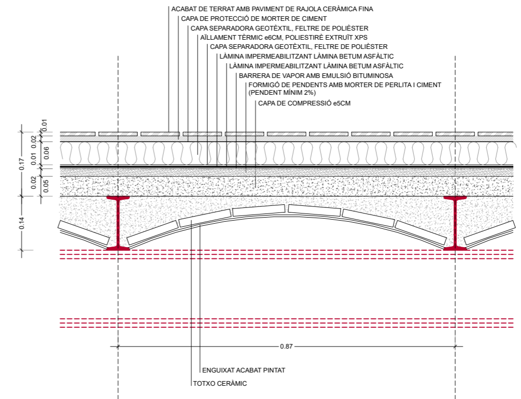
DETALL FORJAT - TERRAT COBERTA PROPOSTA e1/10
