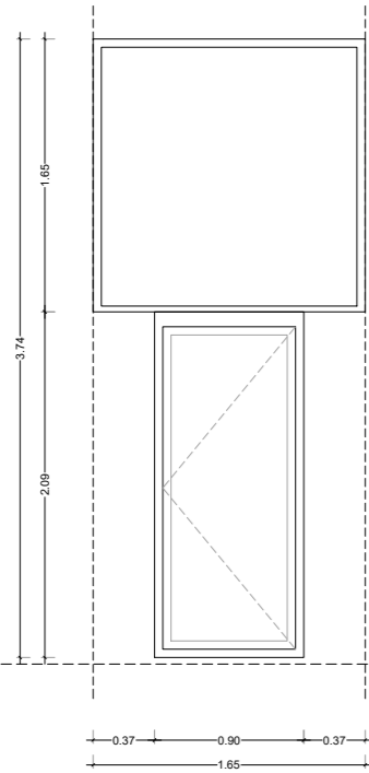
ESTAT ACTUAL FUSTERIA - F01
