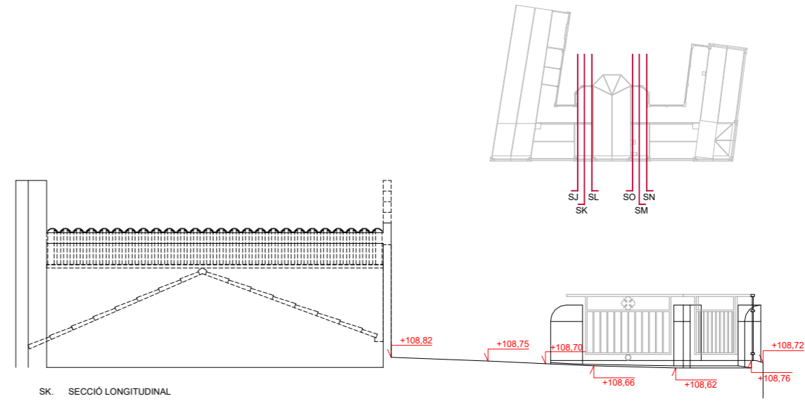
SK. SECCIÓ LONGITUDINAL
