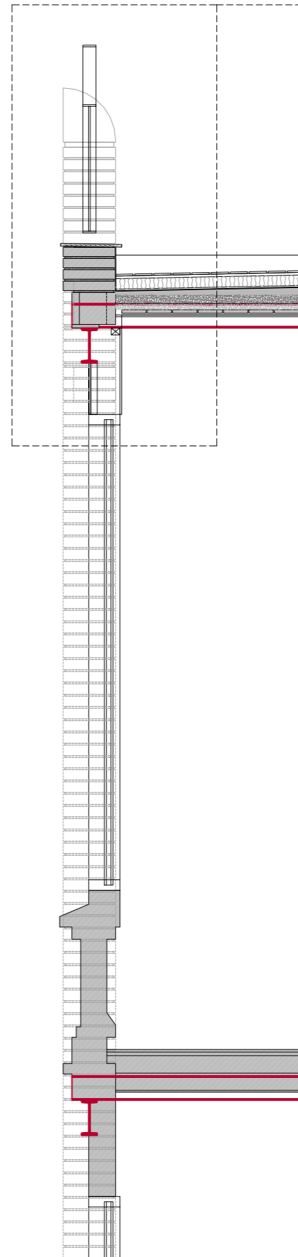
SECCIÓ FAÇANA PATI INTERIOR e1/30
