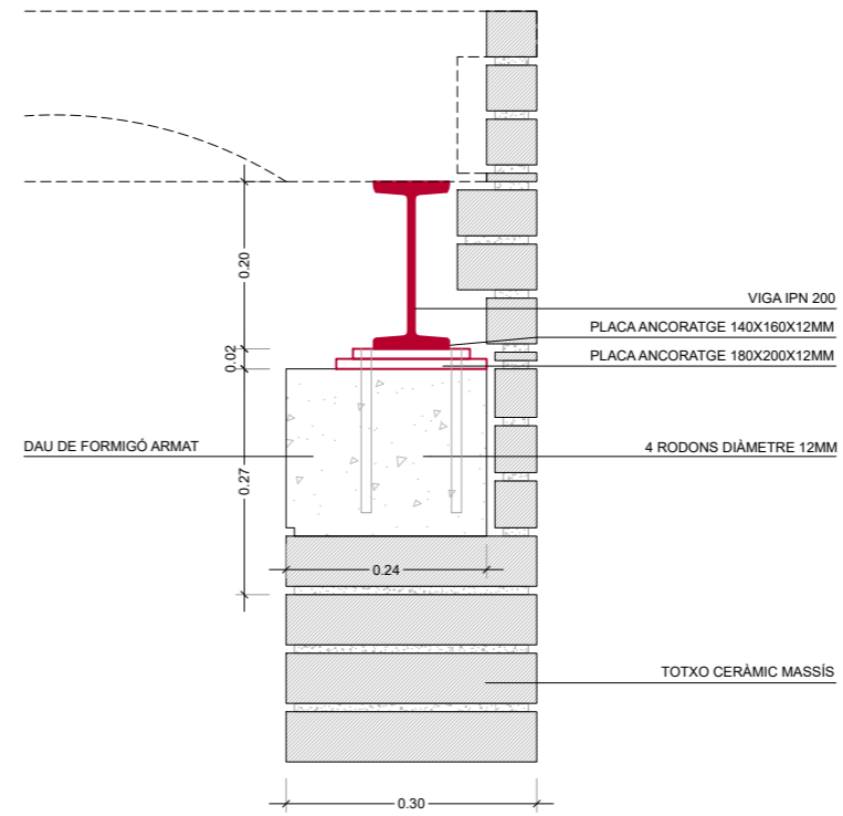
DETALL SECCIÓ 02 - SECCIÓ CAPITELL PILAR e1/10
