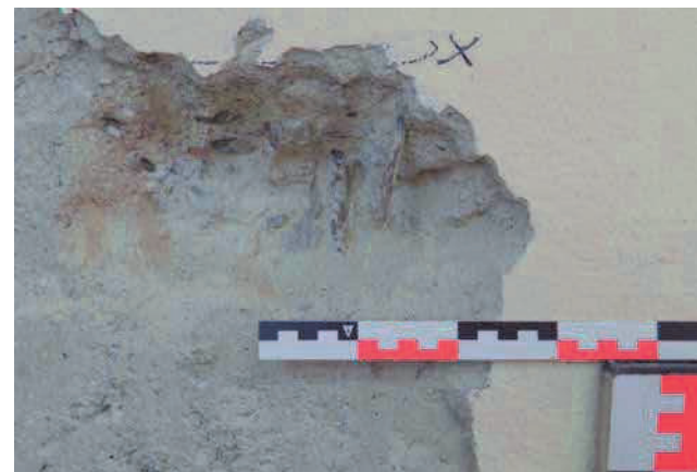
Cala 2.10. Detall on s'observa el ferro de l'armadura
