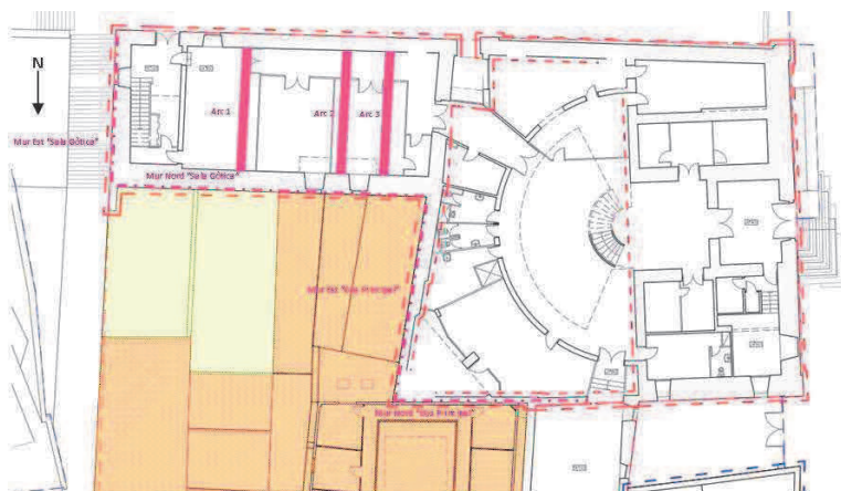
Fig. 8.- Principals elements arquitectònics, històrics i artífics dels Jutjats Vells de Manresa (en rosat).
