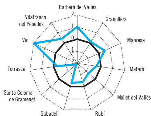
Emissions de CO 2 per habitant*
