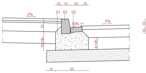
D4 VORADA T2
