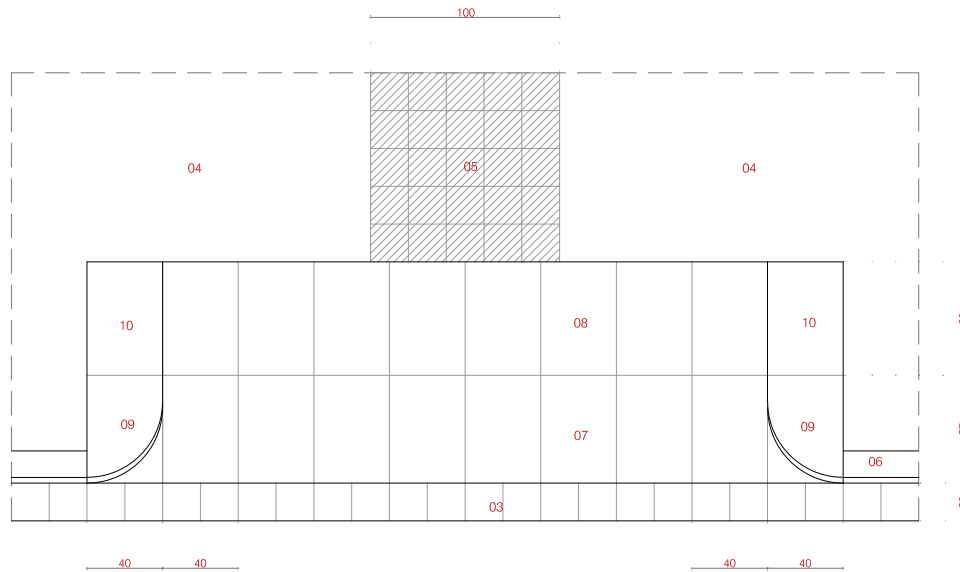
PLANTA
