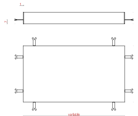
D6 ESCOCELL CIRCULAR/RECTANGULAR D'ACER GALVANITZAT
