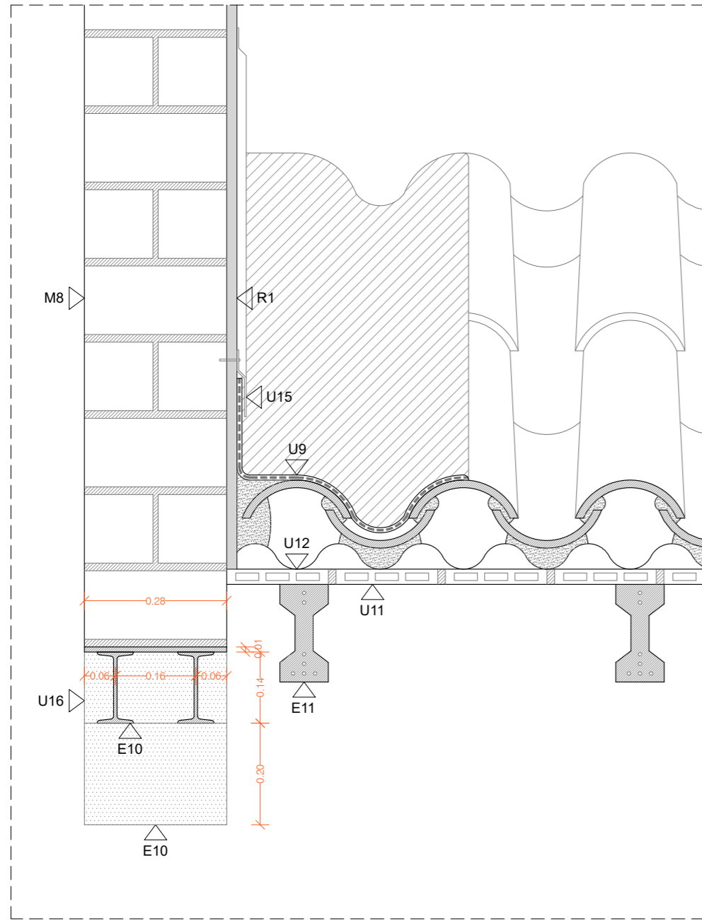
DETALL D07
