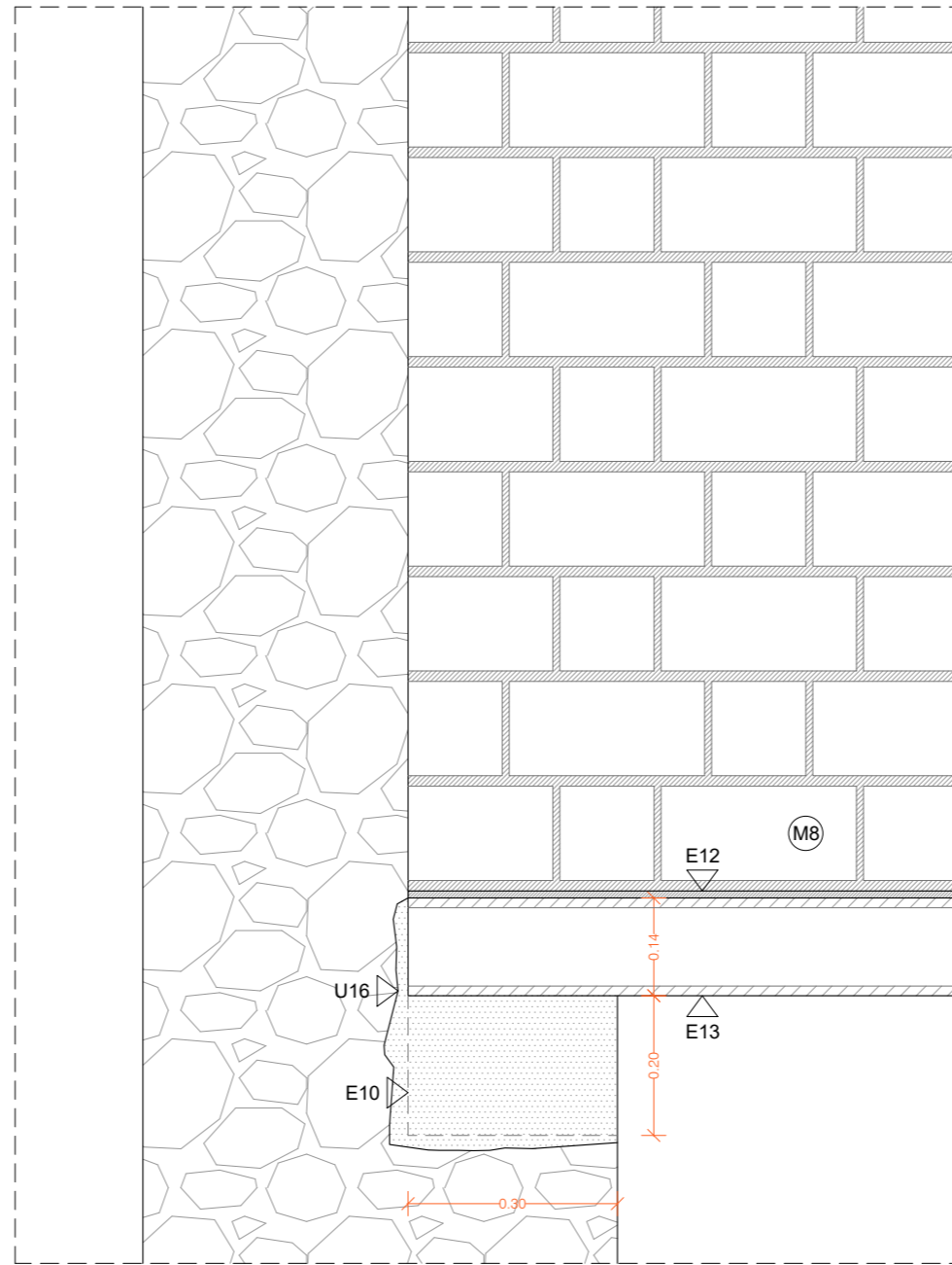
DETALL D08
