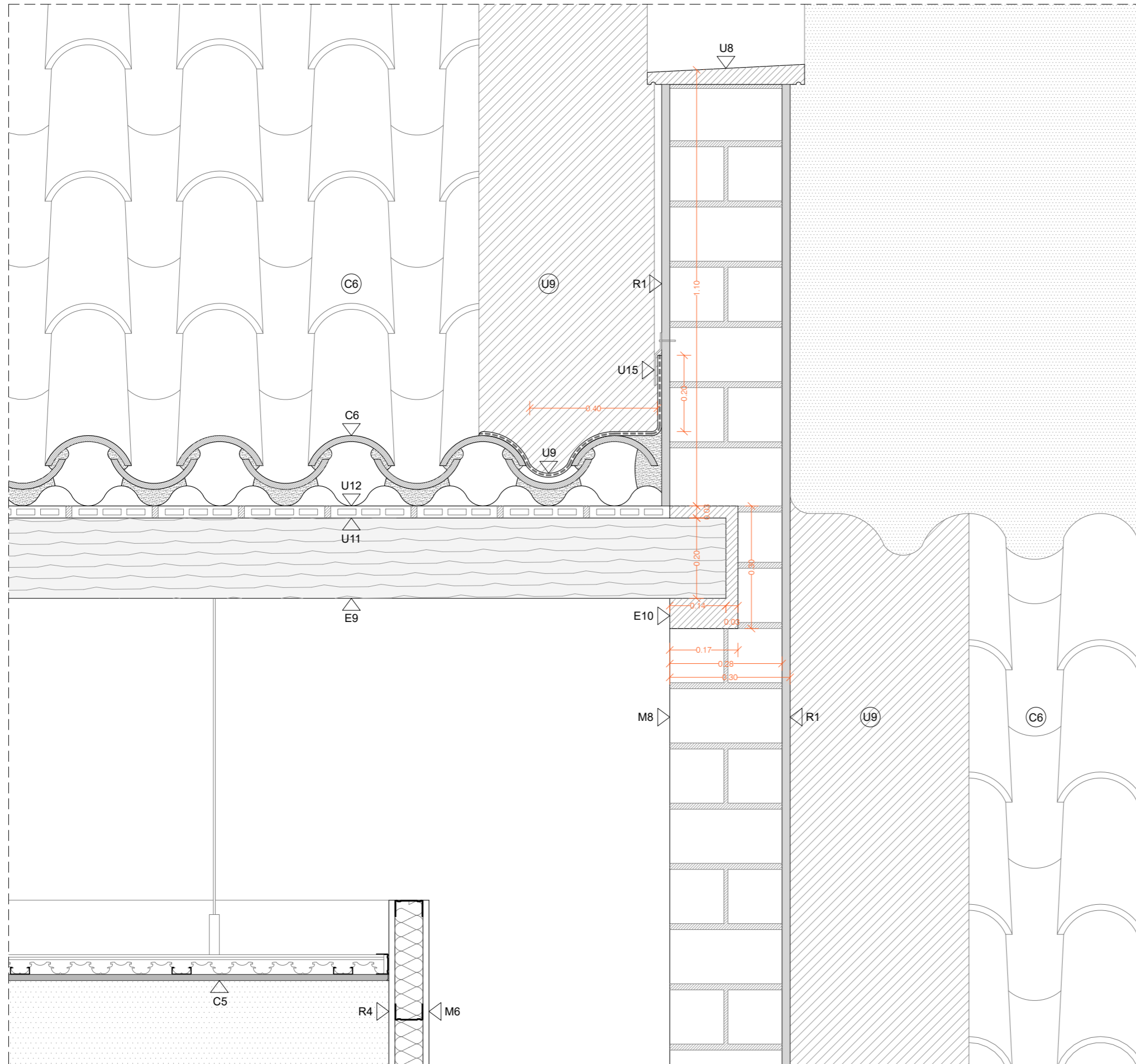
DETALL D03
