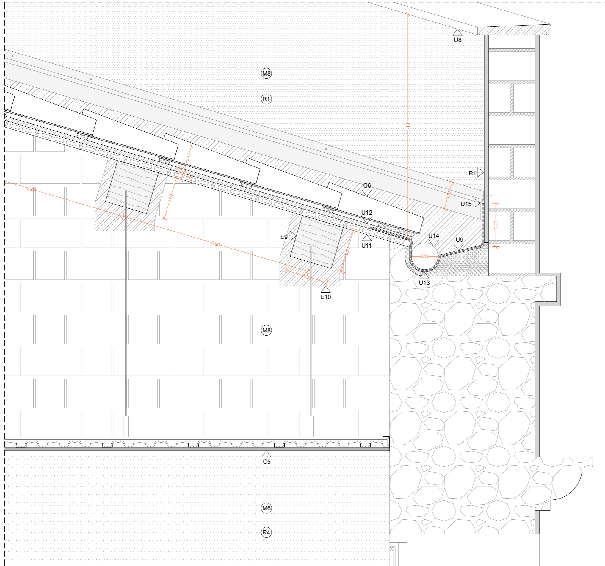
DETALL D01
