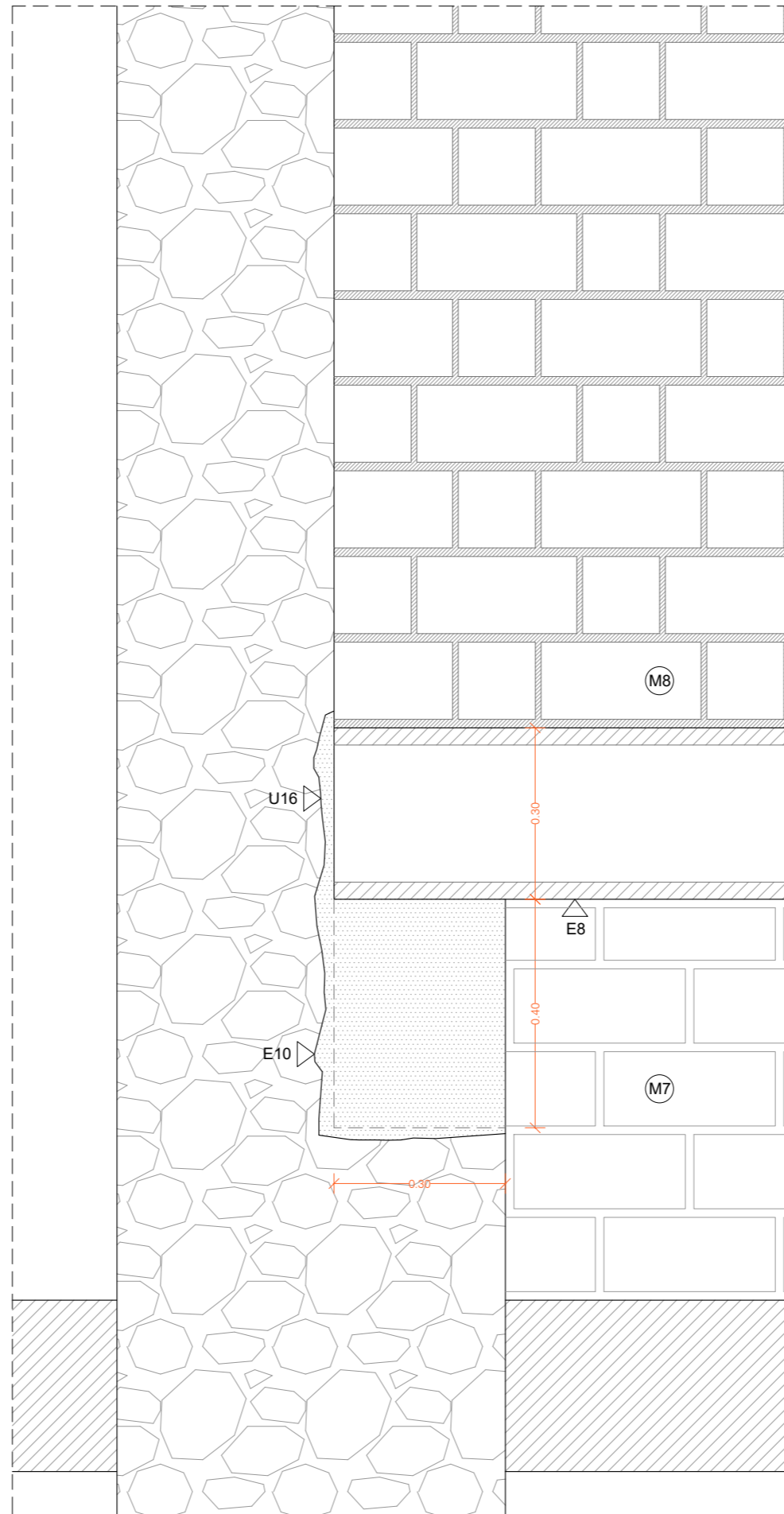
DETALL D06
