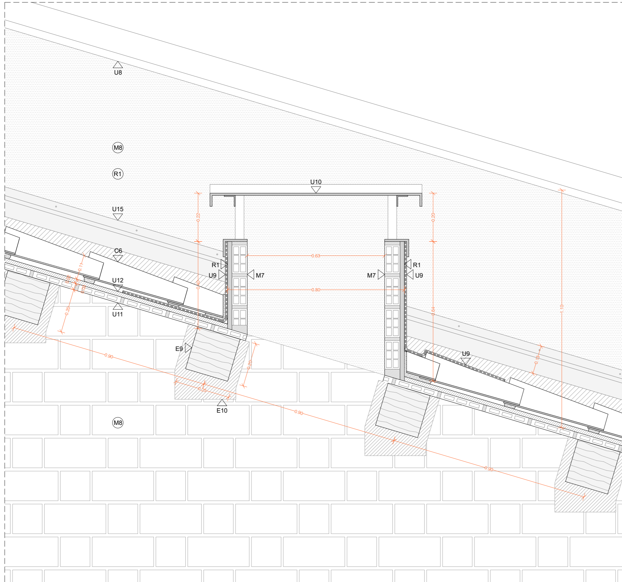
DETALL D02
