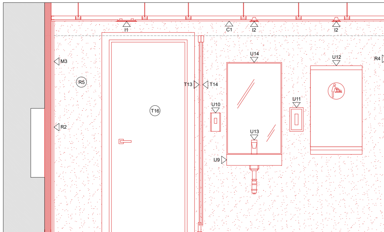
ALÇAT 02
