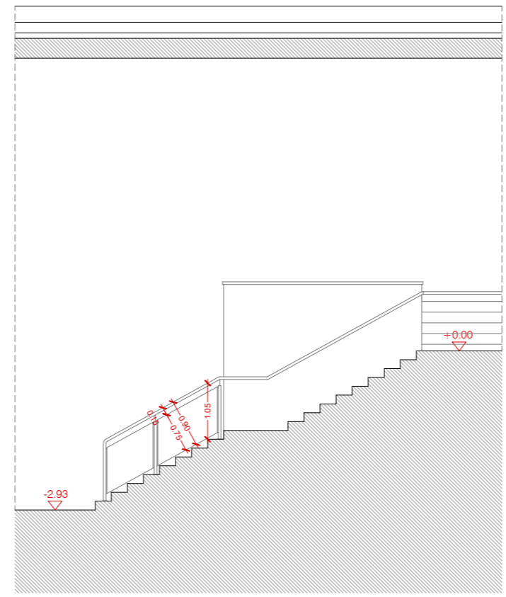
SECCIÓ B-B'
