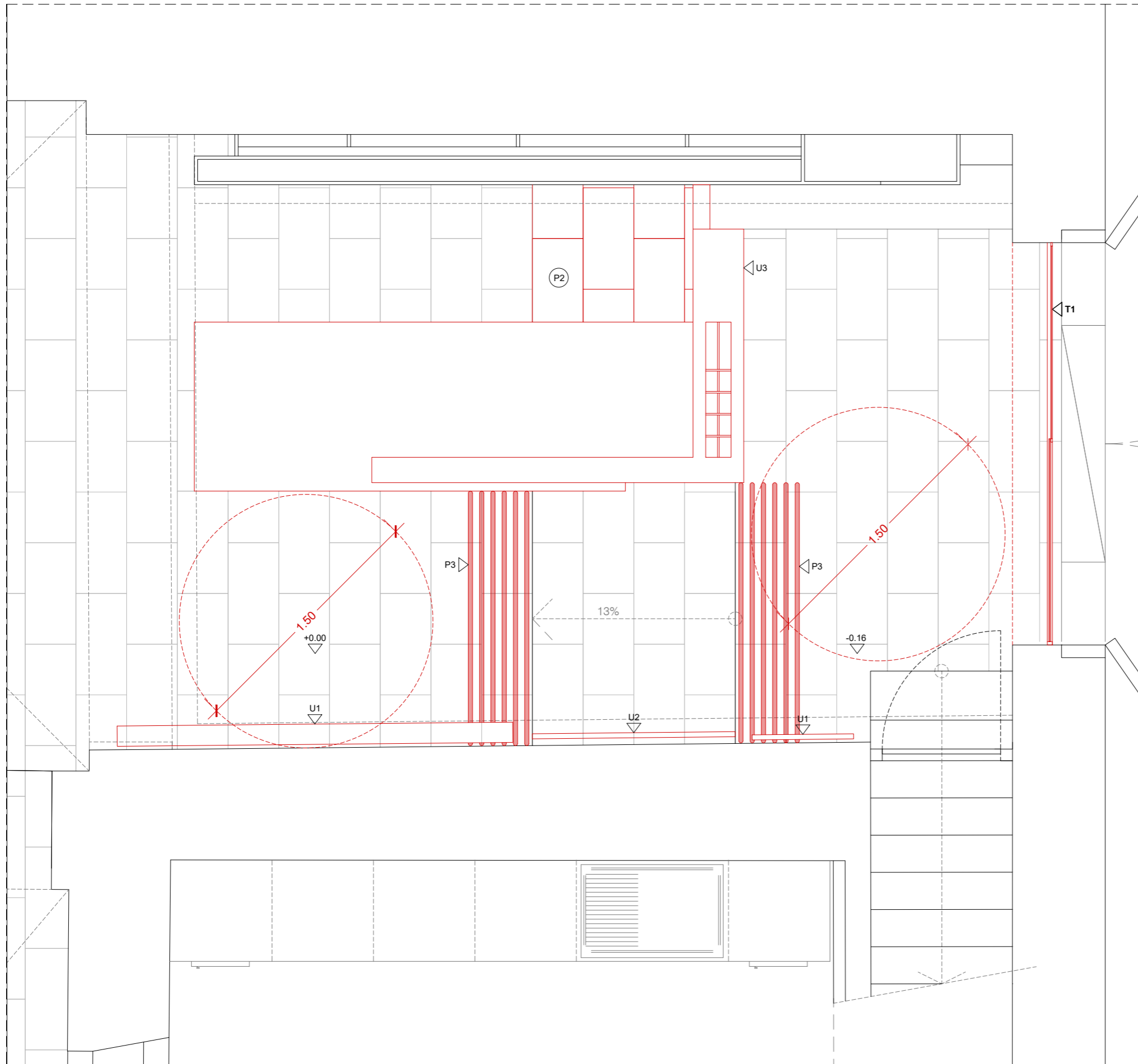
PROPOSTA VESTÍBUL - PLANTA
