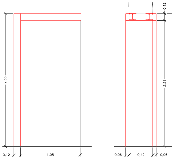
ALÇAT ACCÉS
