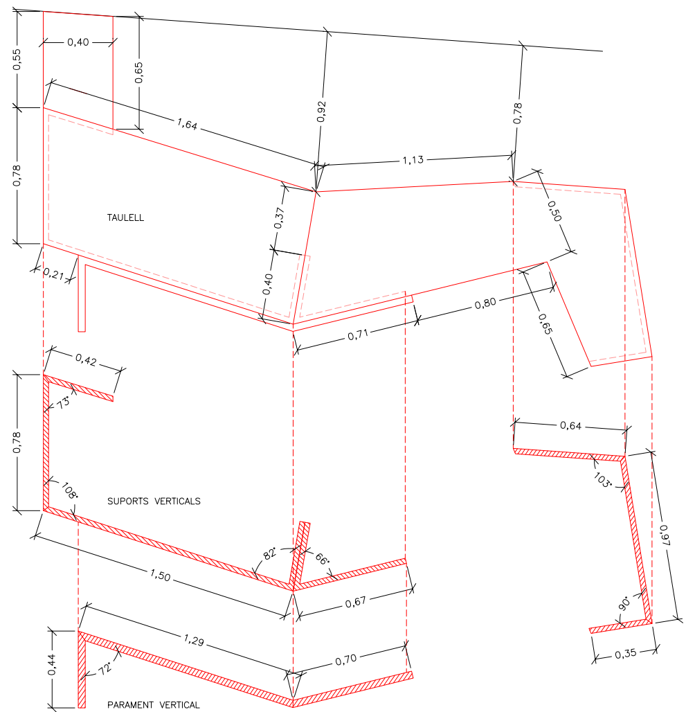
PLANTA ACOTADA PER PECES
