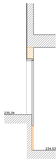
SECCIÓ TRANSVERSAL S1
