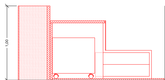
SECCIÓ B-B'
