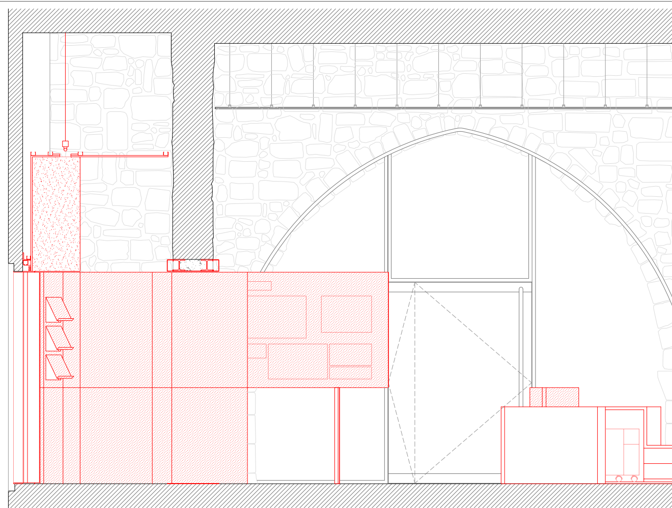
ALÇAT C-C'
