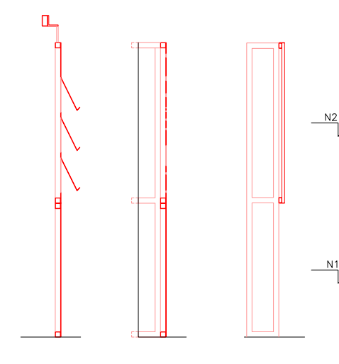
SECCIÓ 1
