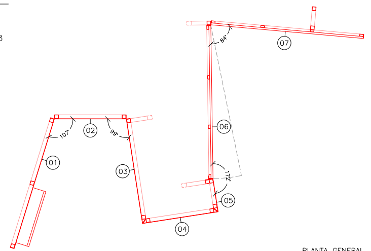
PLANTA GENERAL
