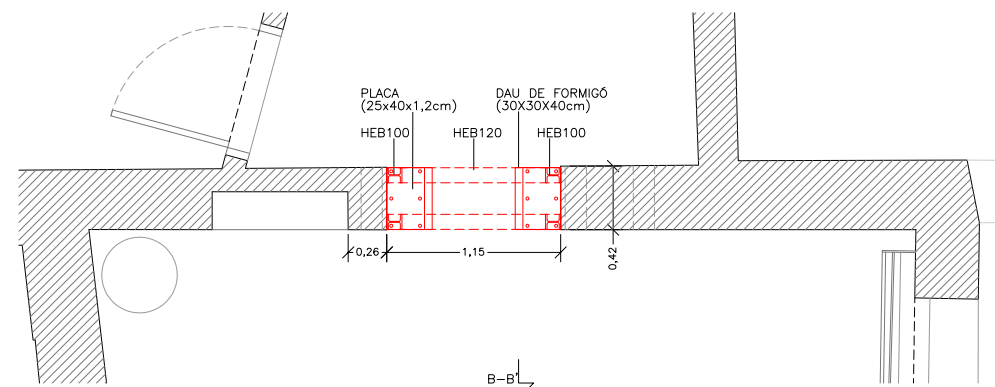
PLANTA PÒRTIC
