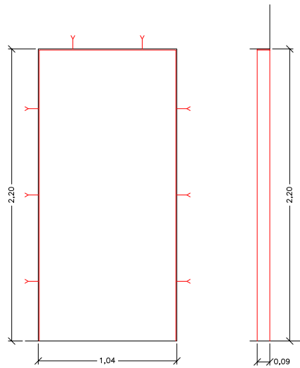
ALÇAT
