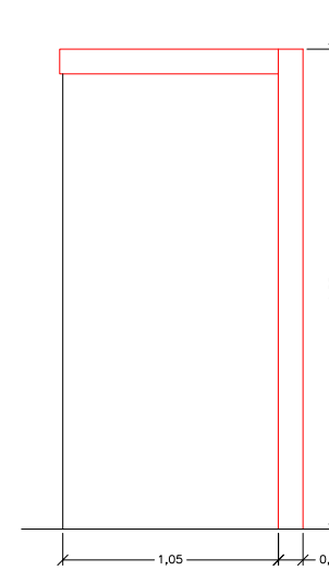
ALÇAT VESTÍBUL ASCENSOR
