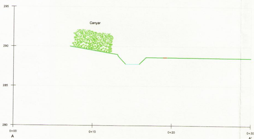
SECCIÓ PK 0+280
