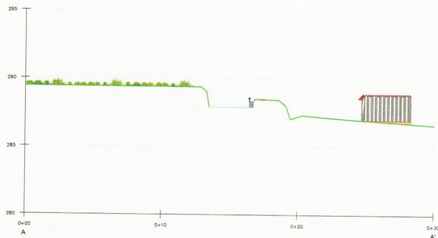
SECCIÓ PK 0+160
