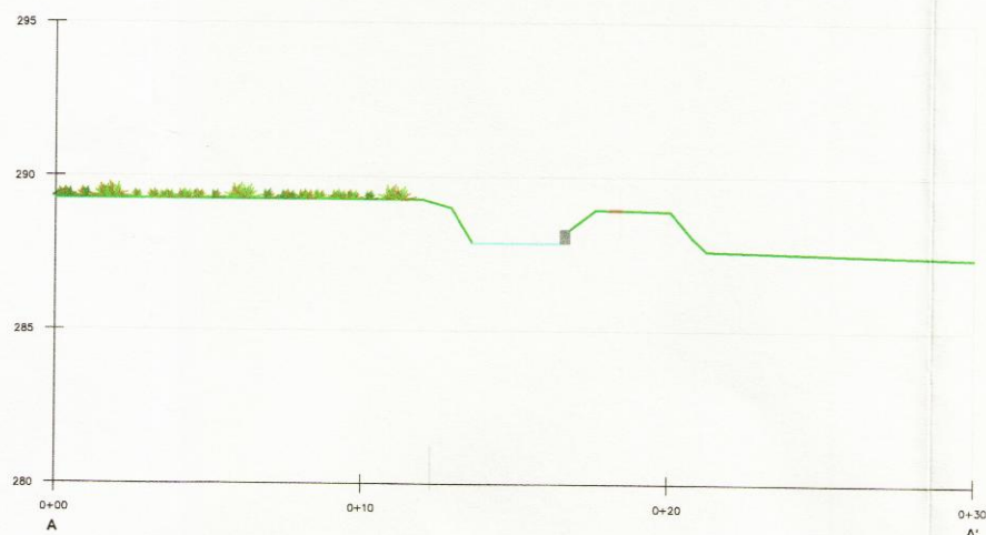
SECCIÓ PK 0+200
