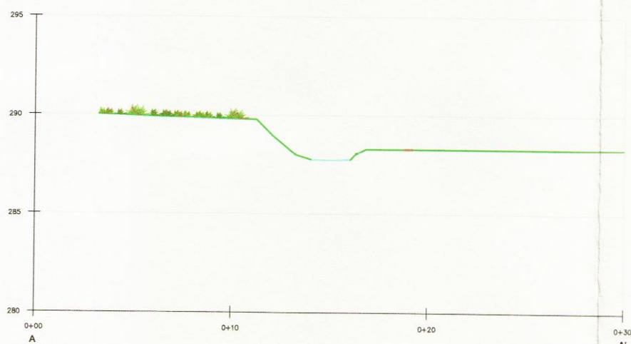
SECCIÓ PK 0+320
