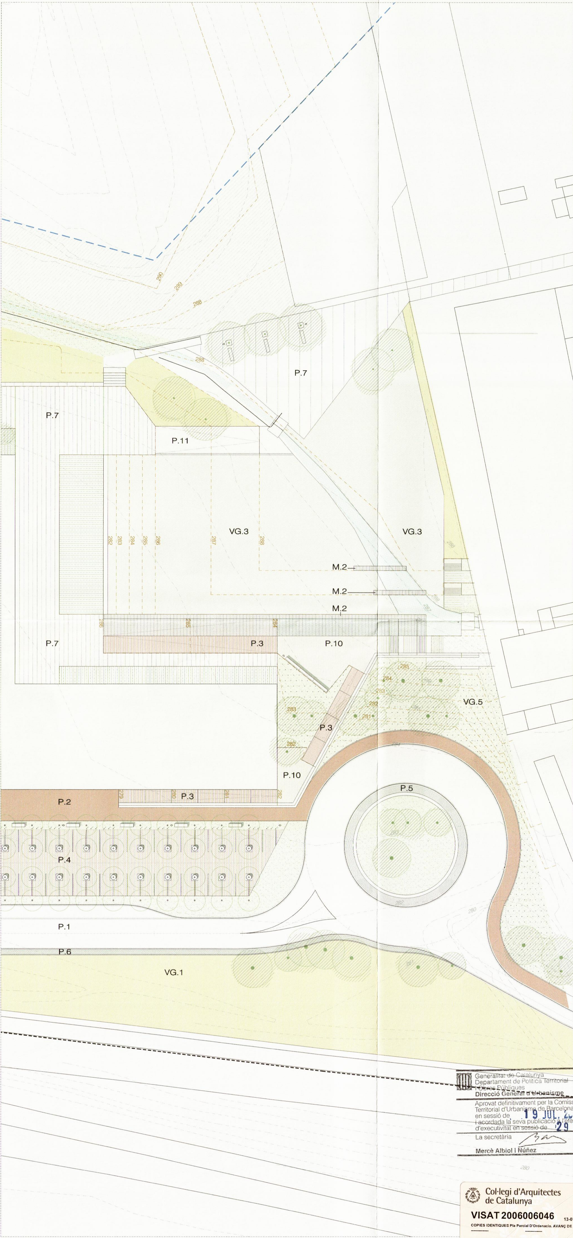
PLANTA P-04
