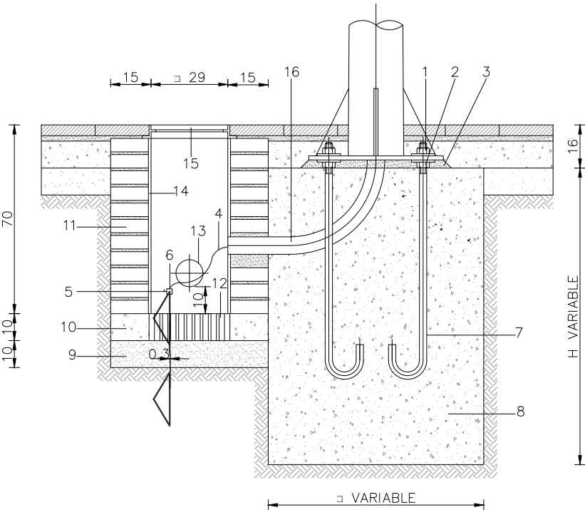
D09 ANCORATGE COLUMNA-ARQUETA
