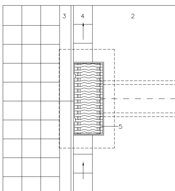
D05 DETALL POU EMBORNAL AMB REIXA TIPUS 'ONDA' LATERAL e: 1/25
