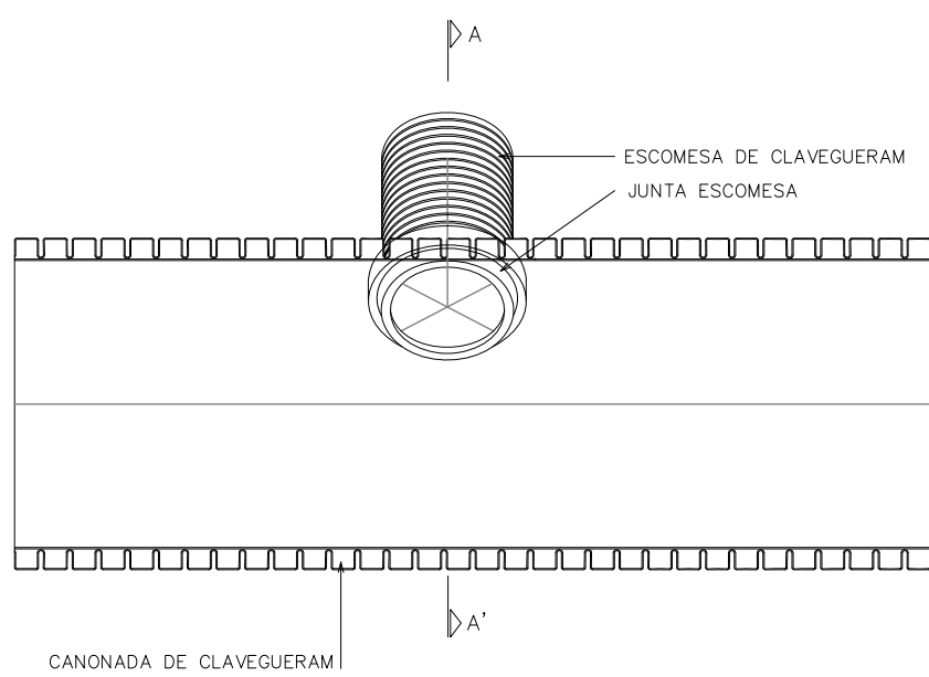
SECCIÓ LONGITUDINAL B-B'
