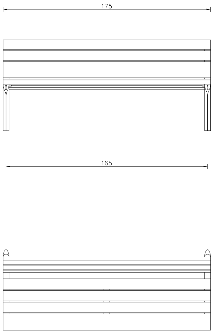
D05 BANC TIPUS NEOROMÀNTIC 175 E: 1/20
