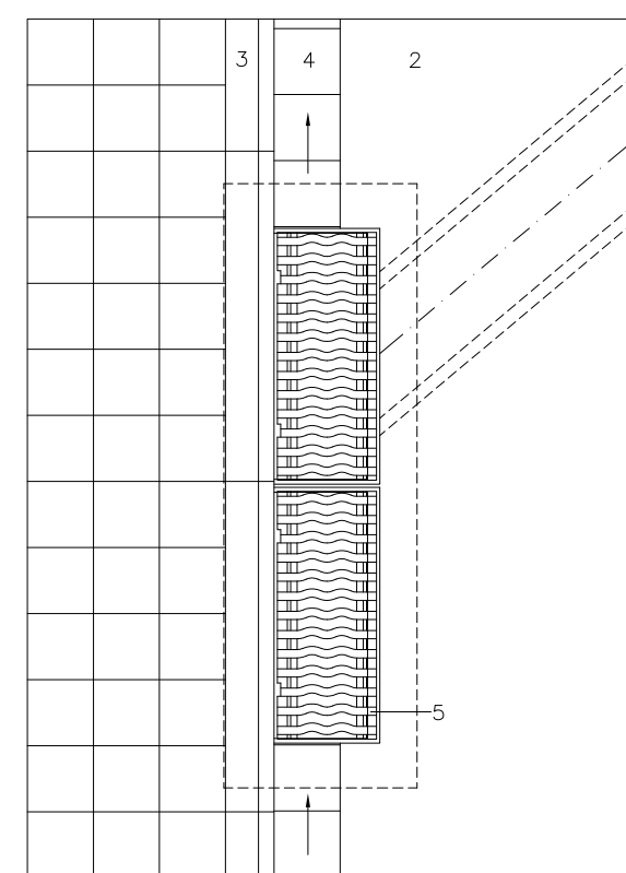
D06 POU EMBORNAL AMB REIXA TIPUS 'ONDA' DOBLE LATERAL e: 1/25
