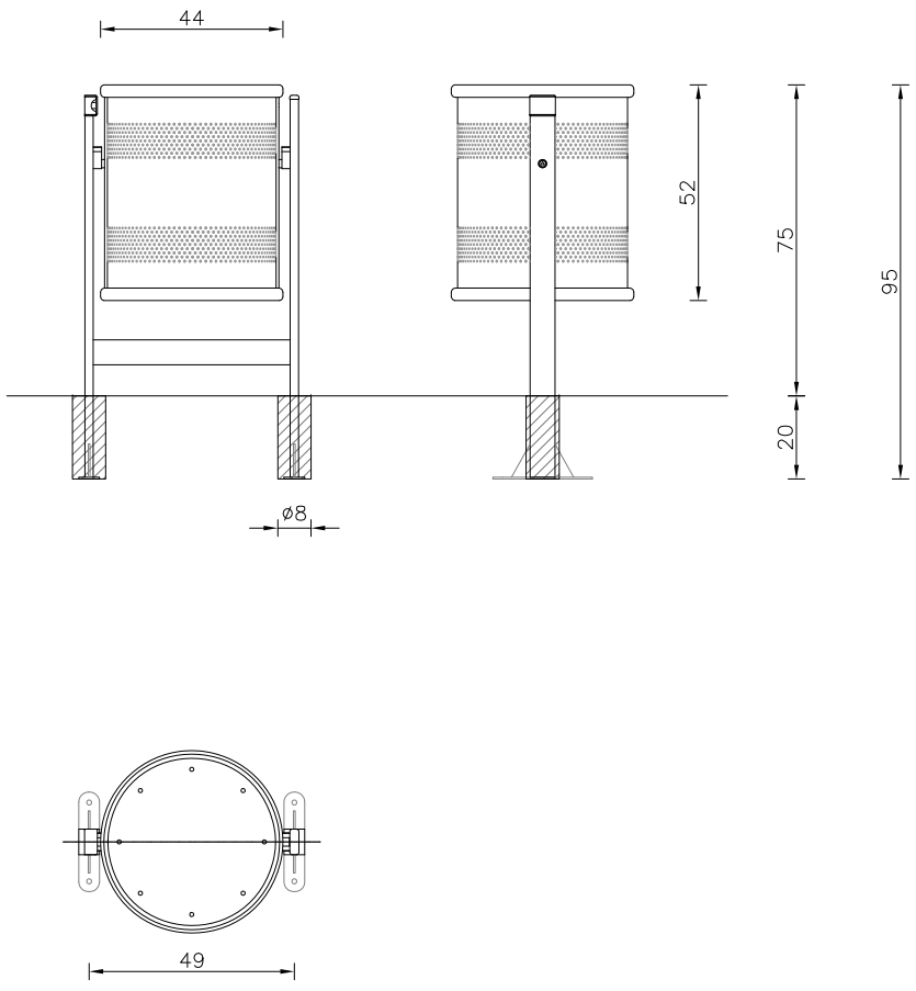
D04 PAPERERA CIRCULAR MODEL BCN DE BENITO E: 1/20
