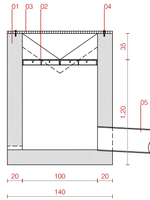
Secció transversal
