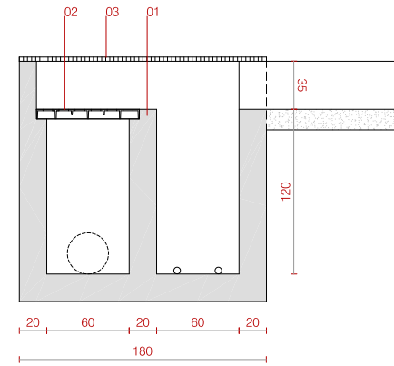
Secció longitudinal
