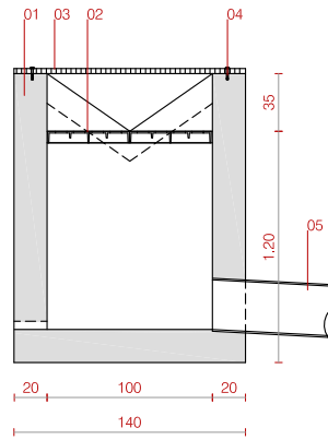
Secció transversal
