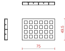
Detall reixa
