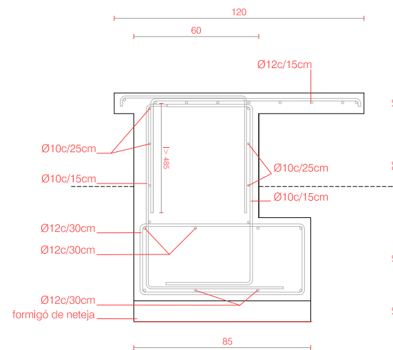
S1. DETALL ARMAT BANC AMB VOLADÍS
