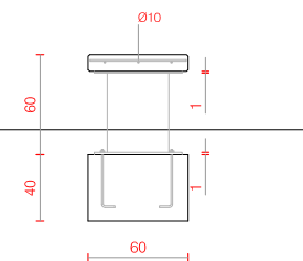
B01 ALÇAT LATERAL BANC
