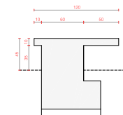
SECCIÓ S1
