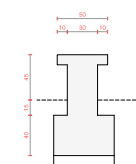
SECCIÓ S2
