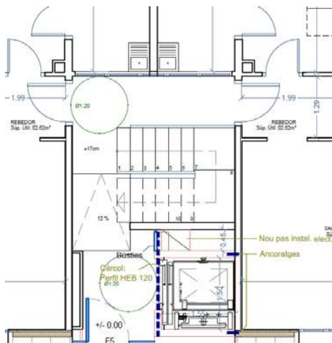
Fig. Planta baixa. Proposta accés.
