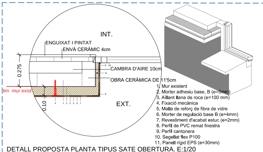
DETALL PROPOSTA PLANTA TIPUS SATE OBERTURA. E: 1/20
