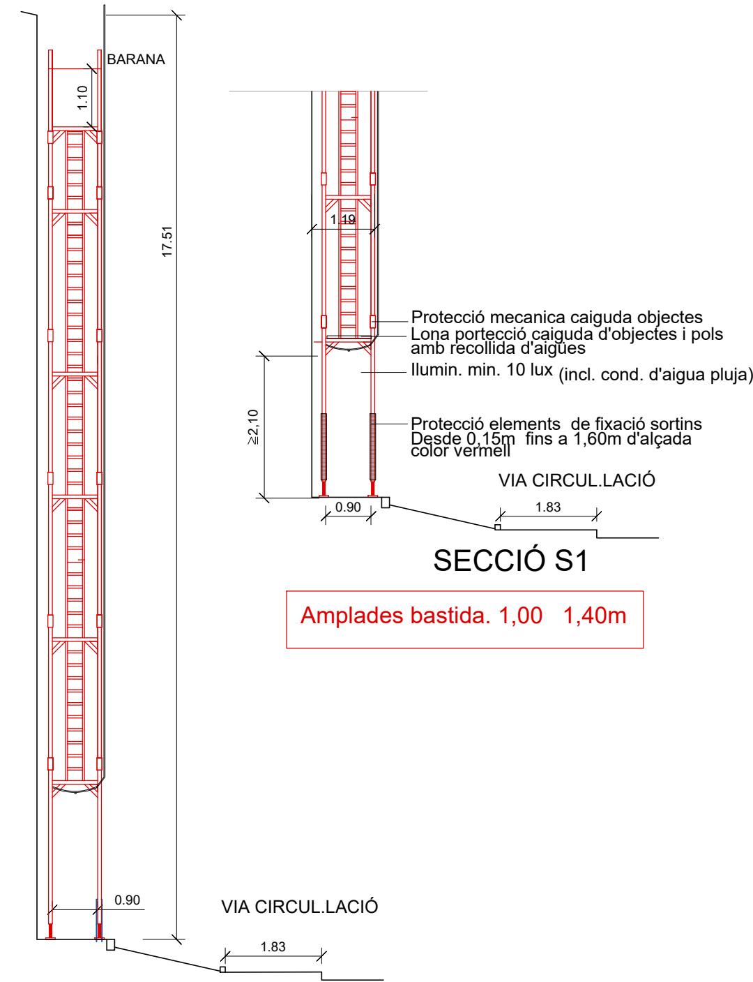
SECCIÓ S1
