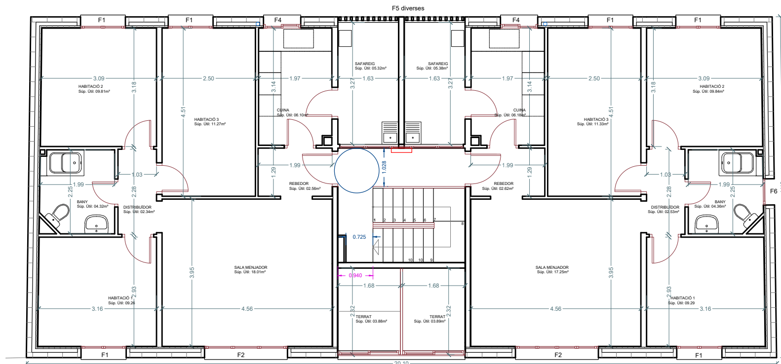
PLANTA PRIMERA
