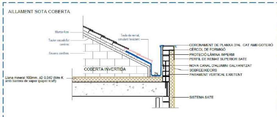
Fig. Detall coberta. Estat projectat.
