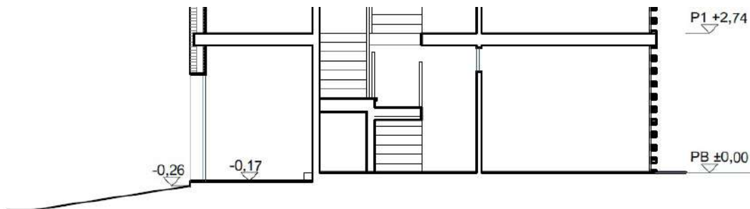
Fig. Secció transversal. Accés actual.
