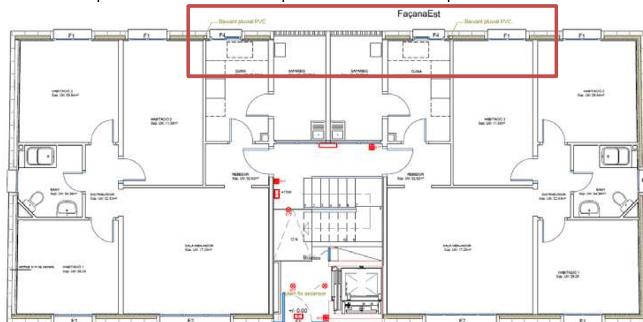
Fig. Planta baixa, ubicació baixants. Estat projectat.
