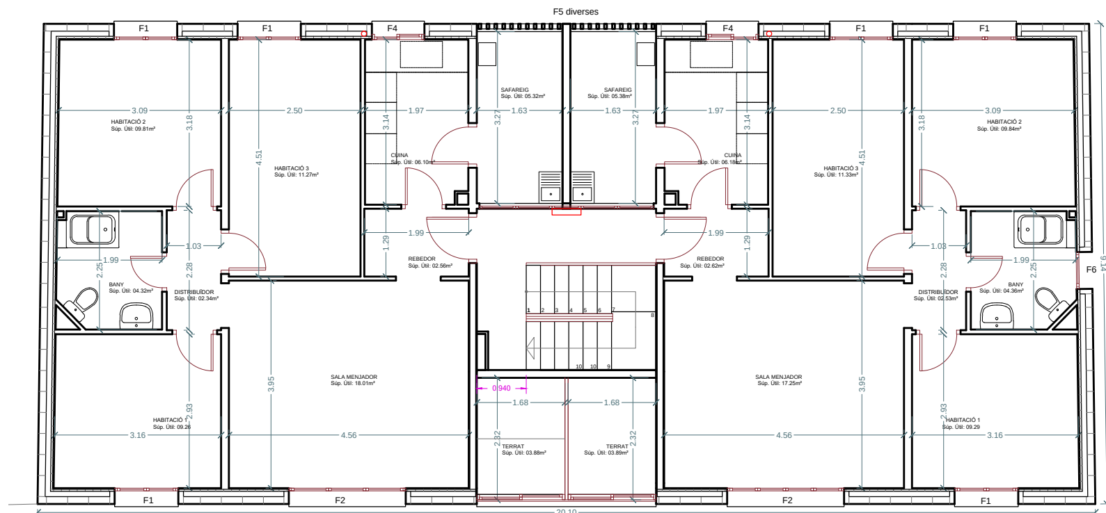
PLANTA PRIMERA
