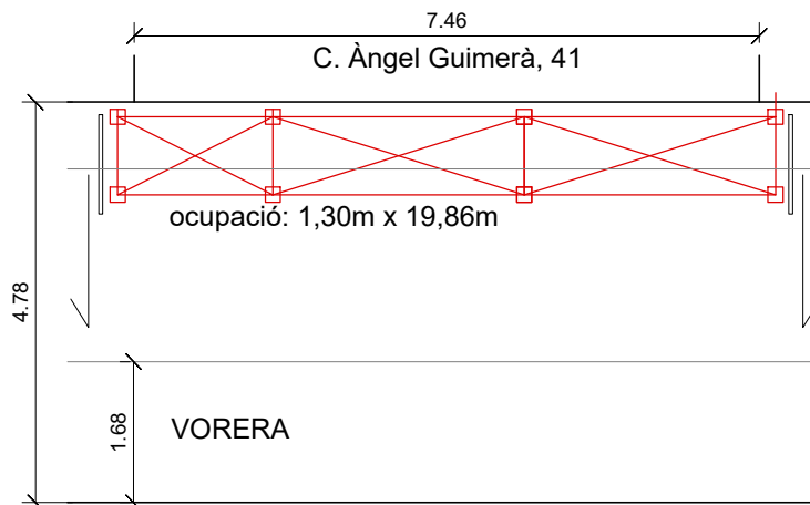
PLANTA
