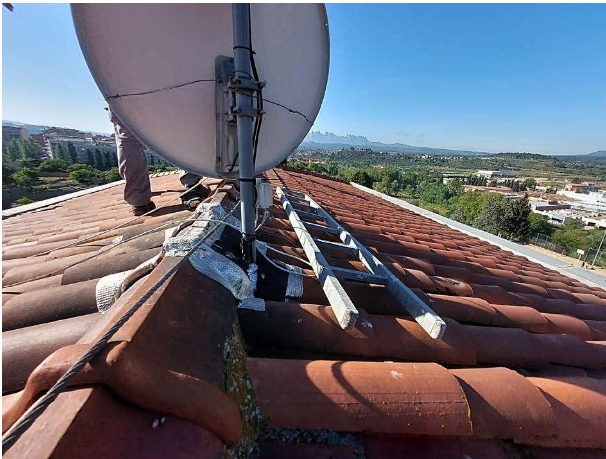
Coberta
