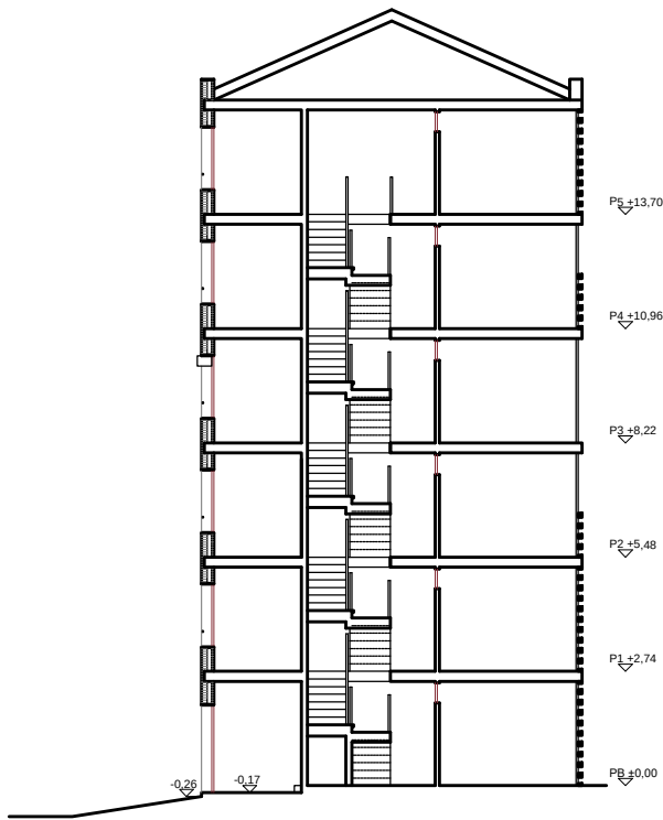
Secció
