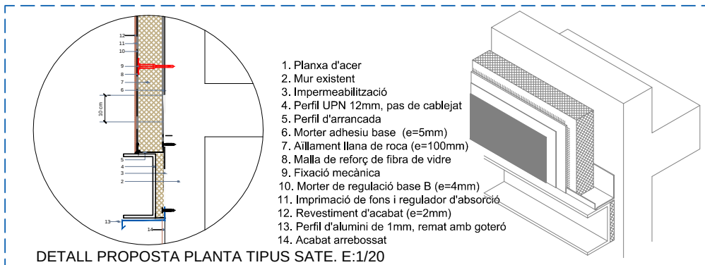
DETALL PROPOSTA PLANTA TIPUS SATE. E: 1/20
