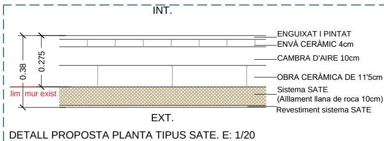
DETALL PROPOSTA PLANTA TIPUS SATE. E: 1/20
