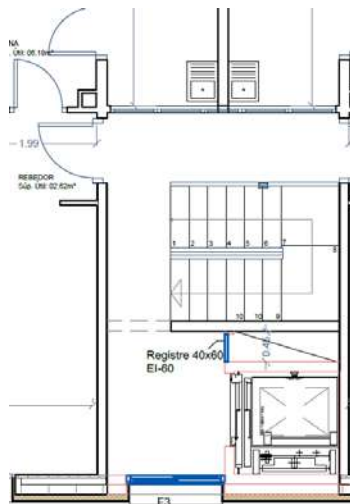
Fig. Planta tipus. Proposta replà.
